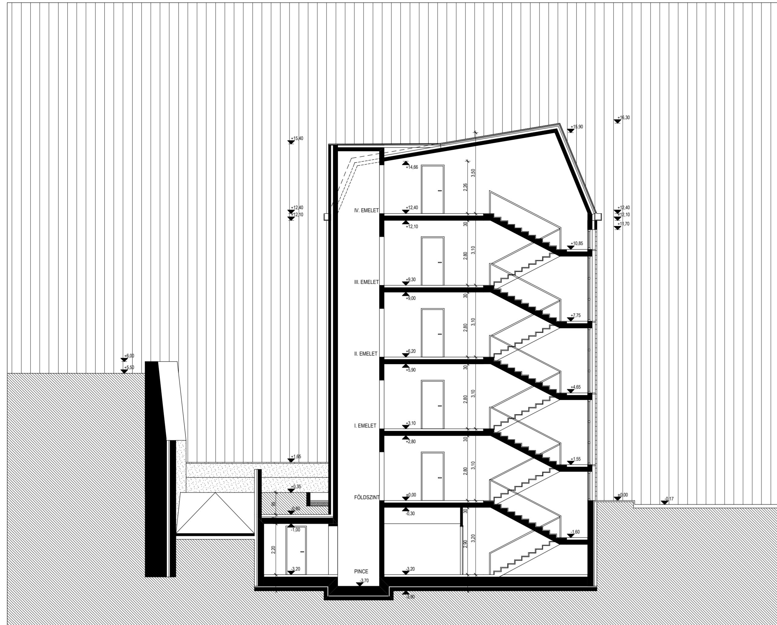
A-A METSZET M 1:100
