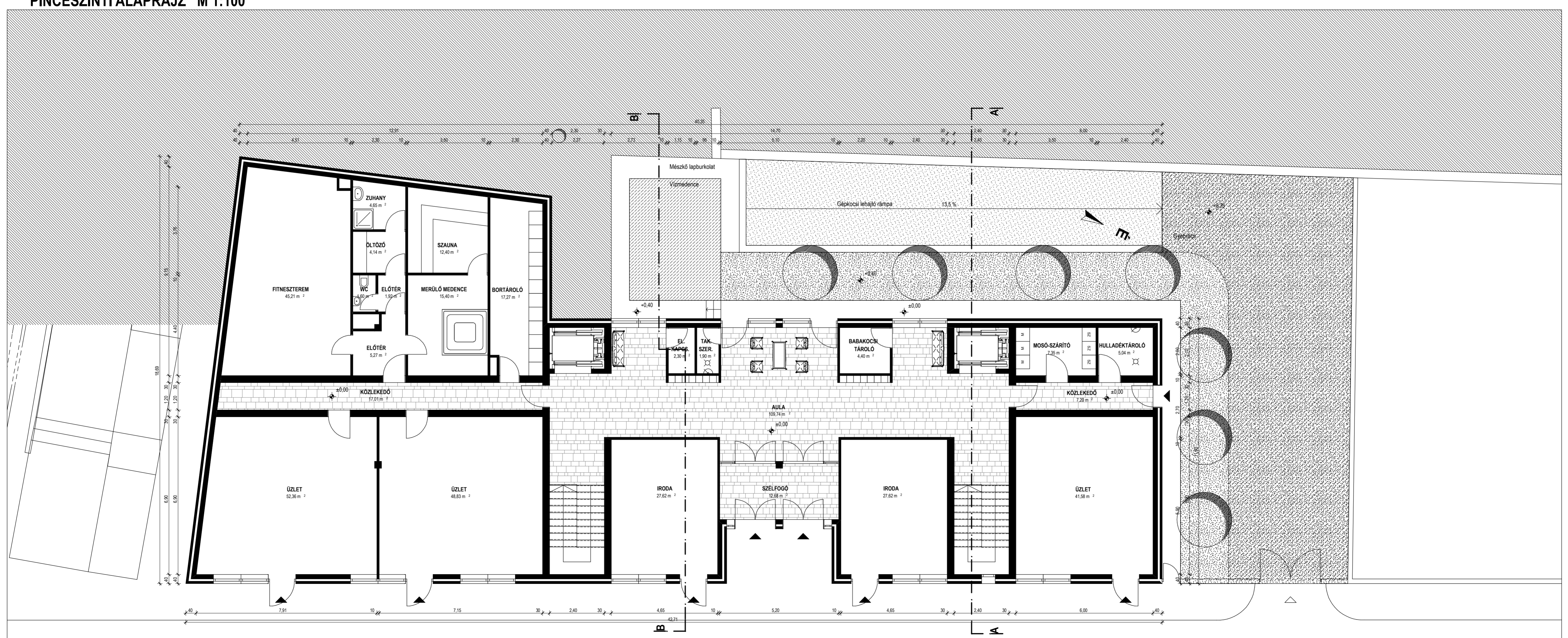
FÖLDSZINTI ALAPRAJZ M 1:100
