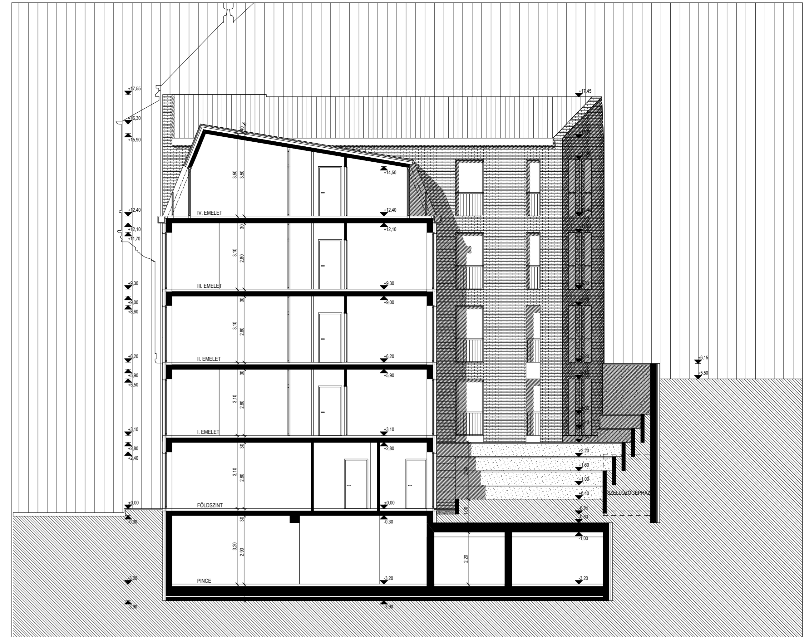
B-B METSZET M 1:100
