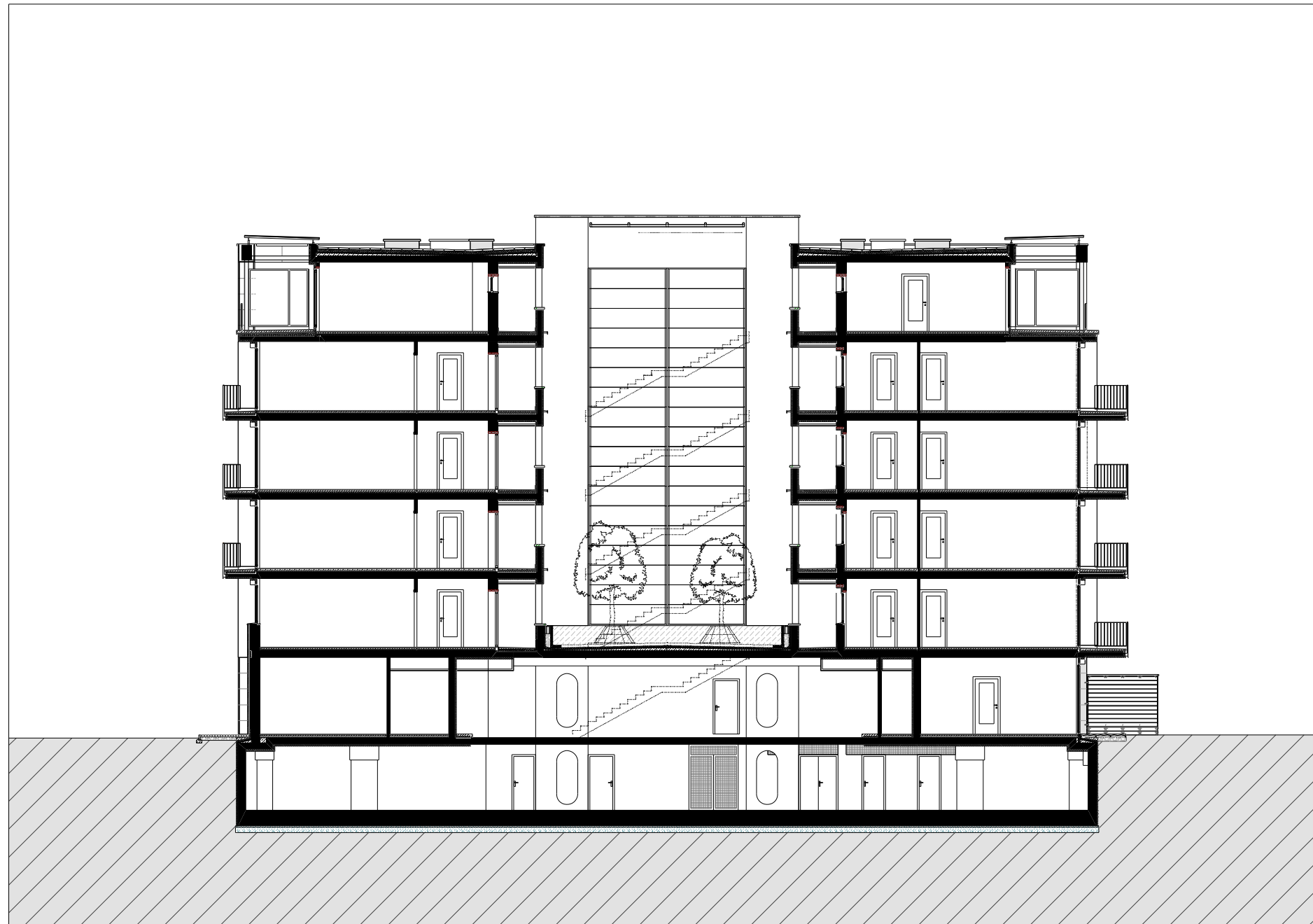
KERESZTMETSZET M1:200
