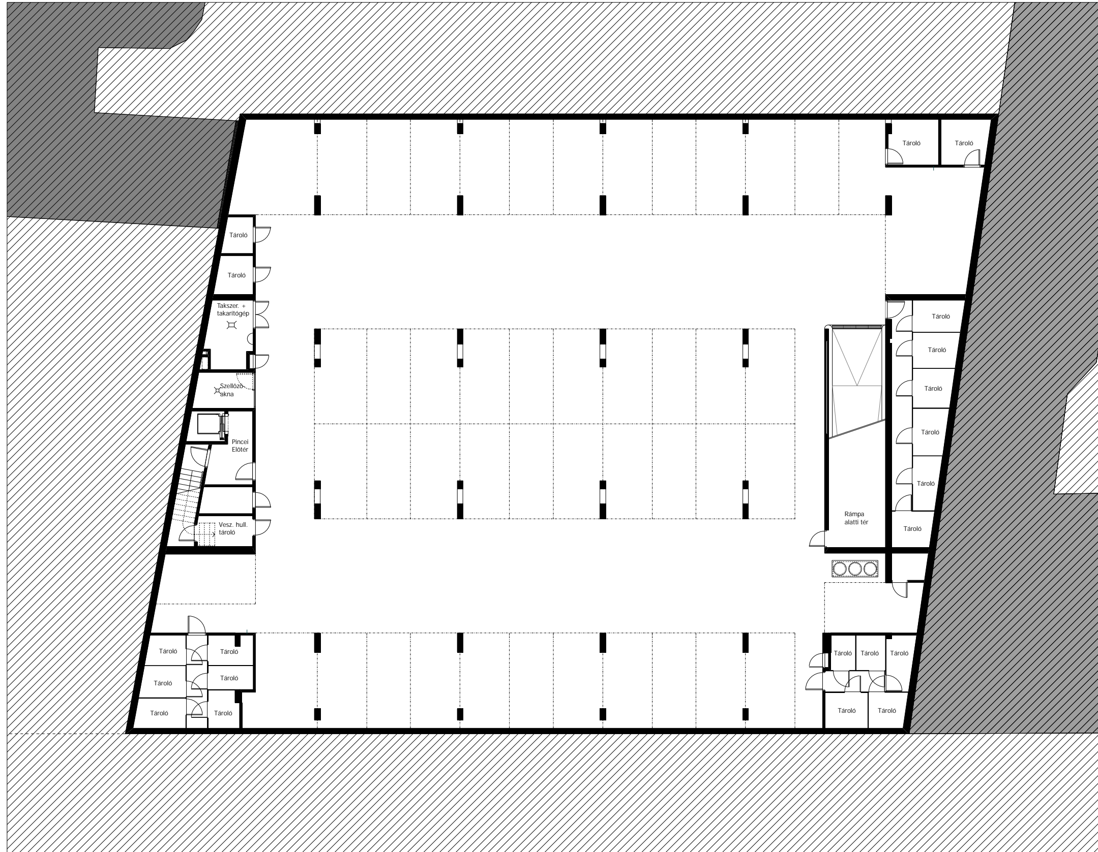
PINCESZINTI ALAPRAJZ M1:200
