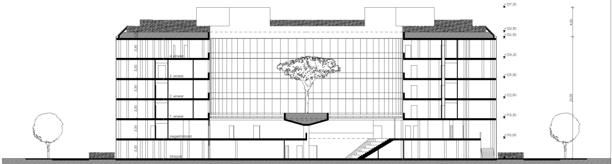
A-A METSZET
