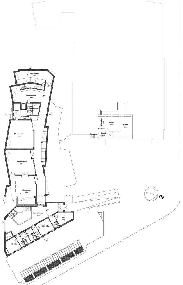
alagsori szint m.1.200
