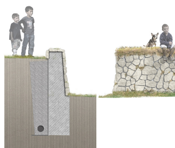
RÉSZLETRAJZOK -- M 1:20
