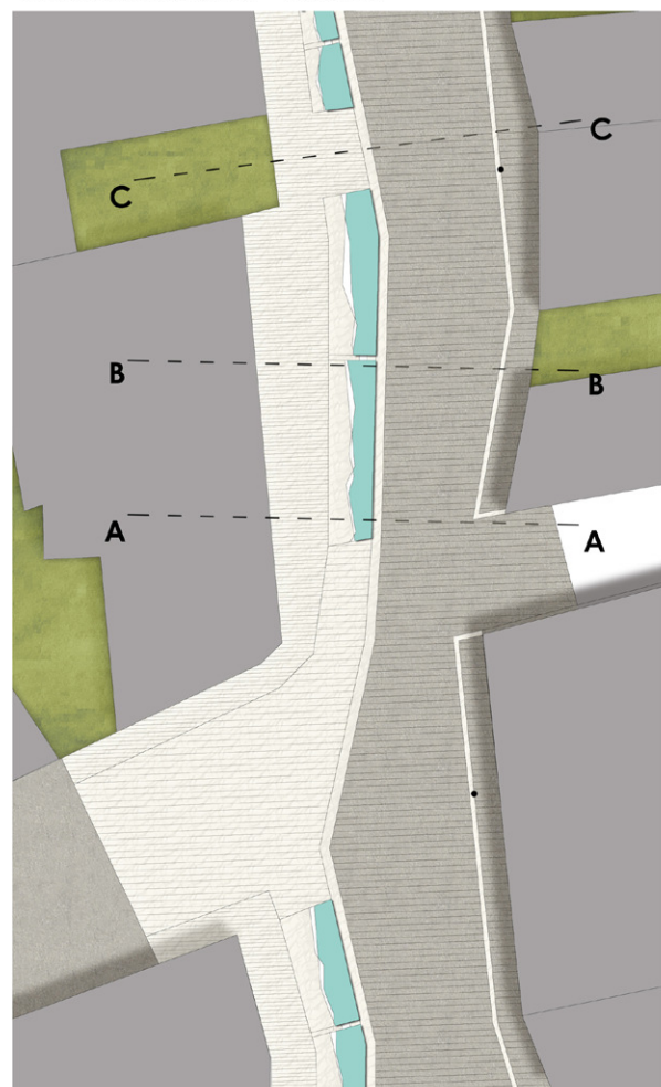
VINCE UTCA RÉSZLETE -- M 1:200
