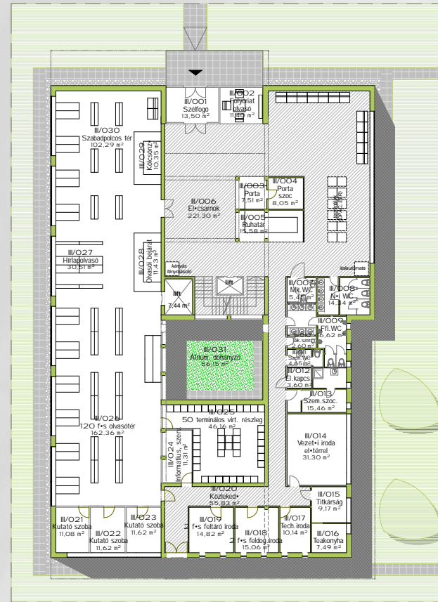
Földszinti alaprajz
