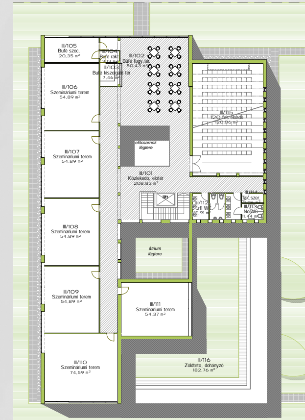
Emeleti alaprajz
