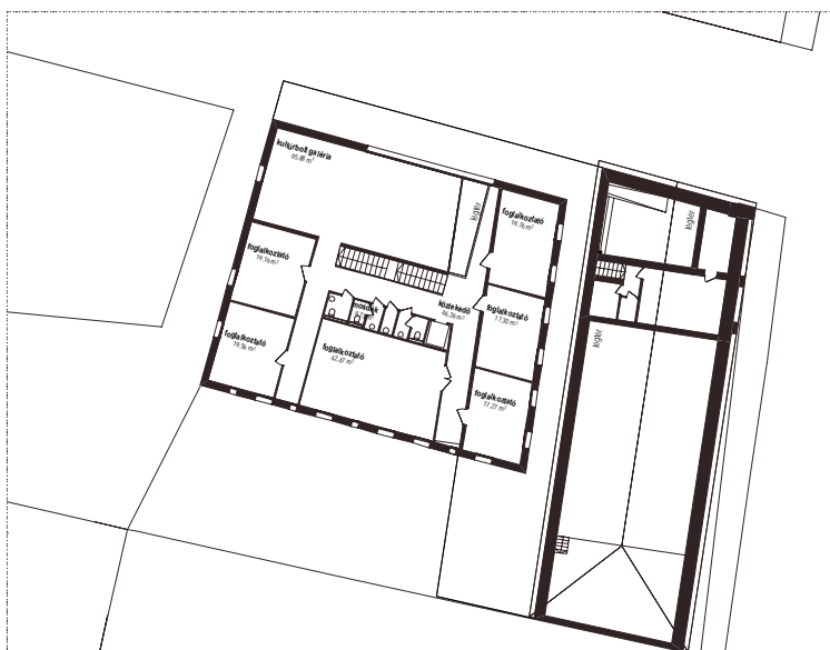
MOZI ÉS MŰVELŐDÉSI HÁZ, ÁTALAKÍTÁS, EMELETI ALAPRAJZ M 1:200
