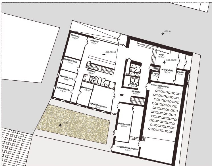
MOZI ÉS MŰVELŐDÉSI HÁZ, ÁTALAKÍTÁS, FÖLDSZINTI ALAPRAJZ M 1:200
