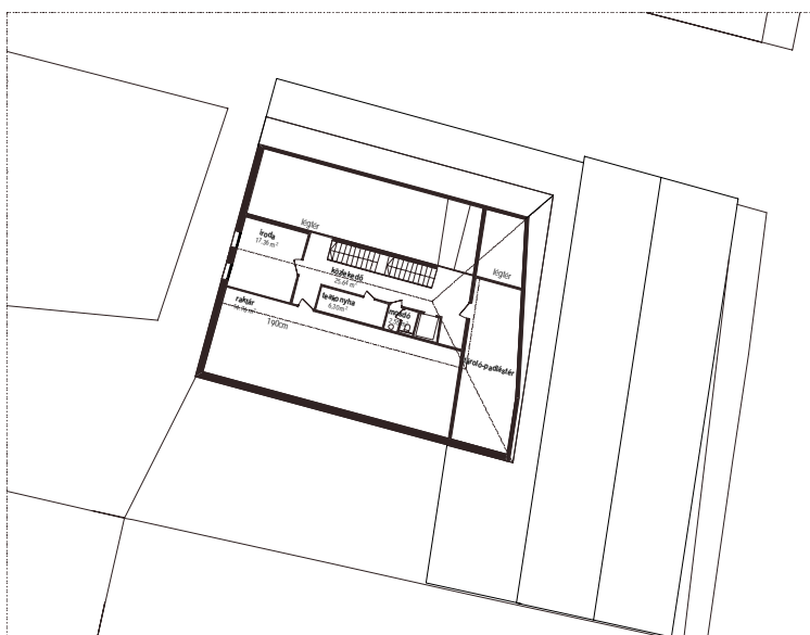
MOZI ÉS MŰVELŐDÉSI HÁZ, ÁTALAKÍTÁS, TETŐTÉRI ALAPRAJZ M 1:200
