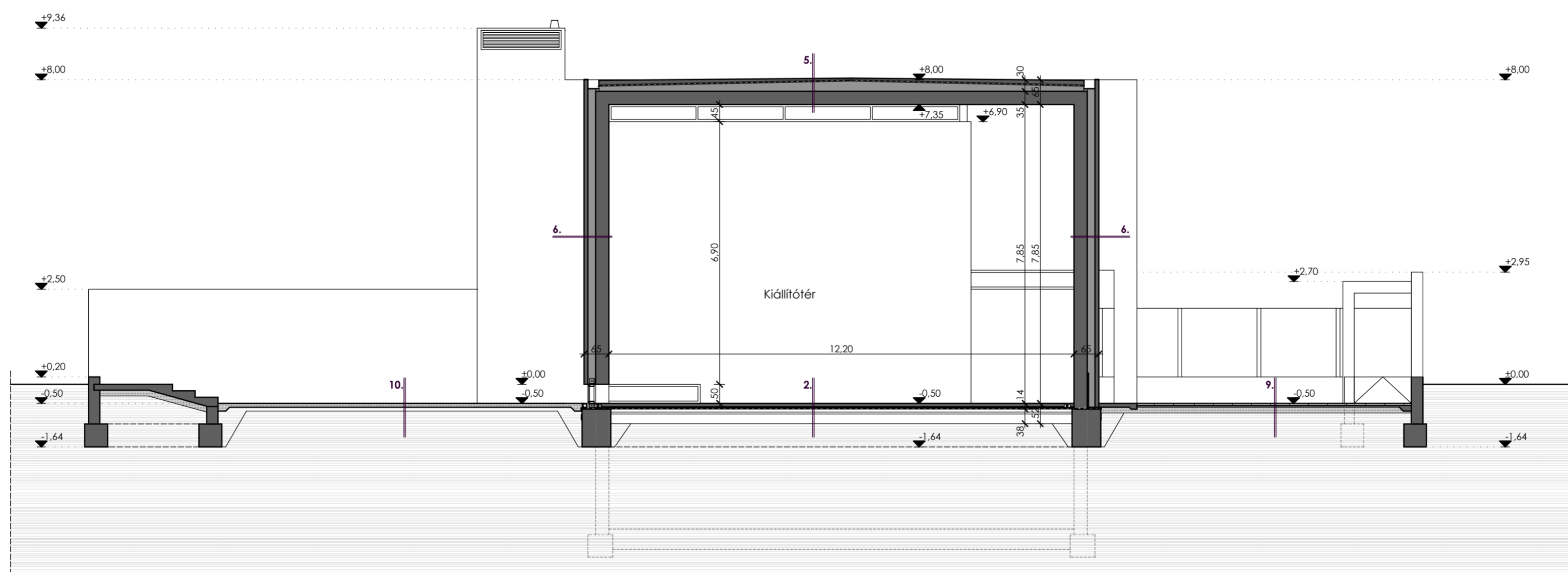
D-D METSZET
