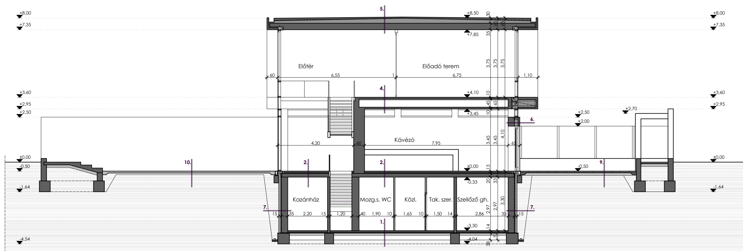
C-C METSZET
