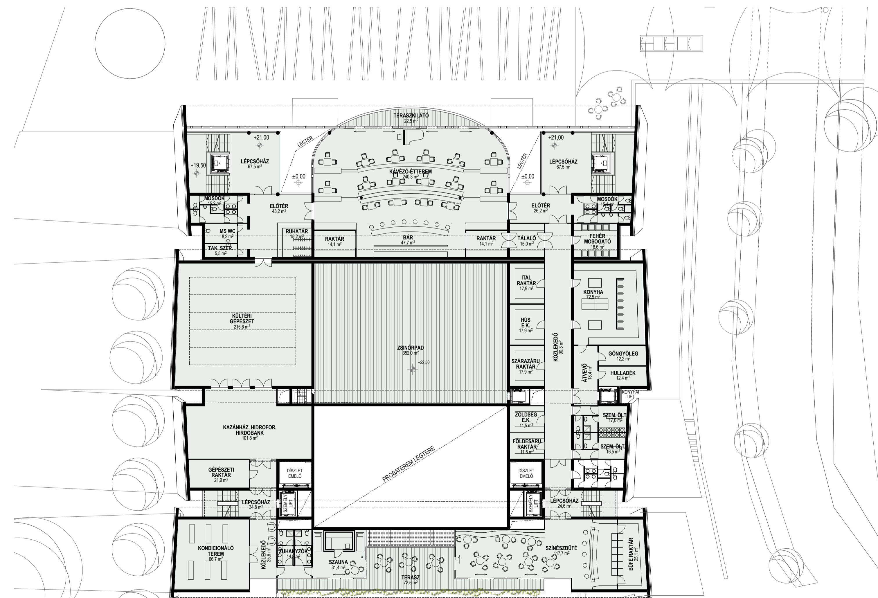
VI. EMELETI ALAPRAJZ +18,00m M=1:250
