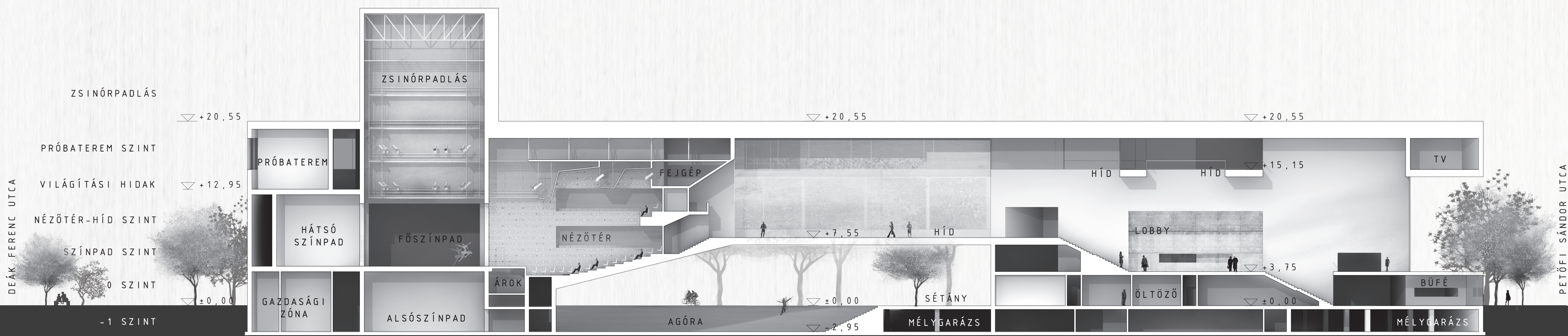
2-2 METSZET M 1:250
