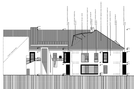
ÉSZAKKELETI HOMLOKZAT_utcafront
