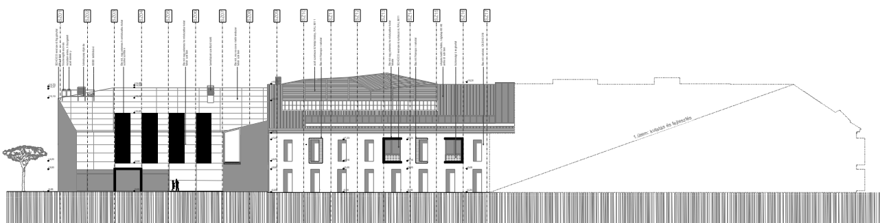
ÉSZAKNYUGATI HOMLOKZAT_belső udvar
