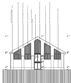
DÉLKELETI HOMLOKZAT_rendezvénytér
