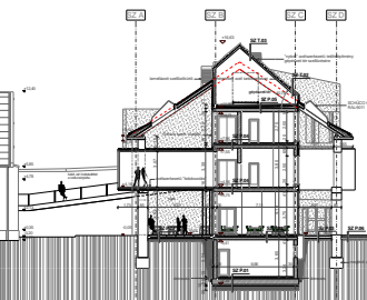
3 - 3 METSZET_kutatói szálláshely
