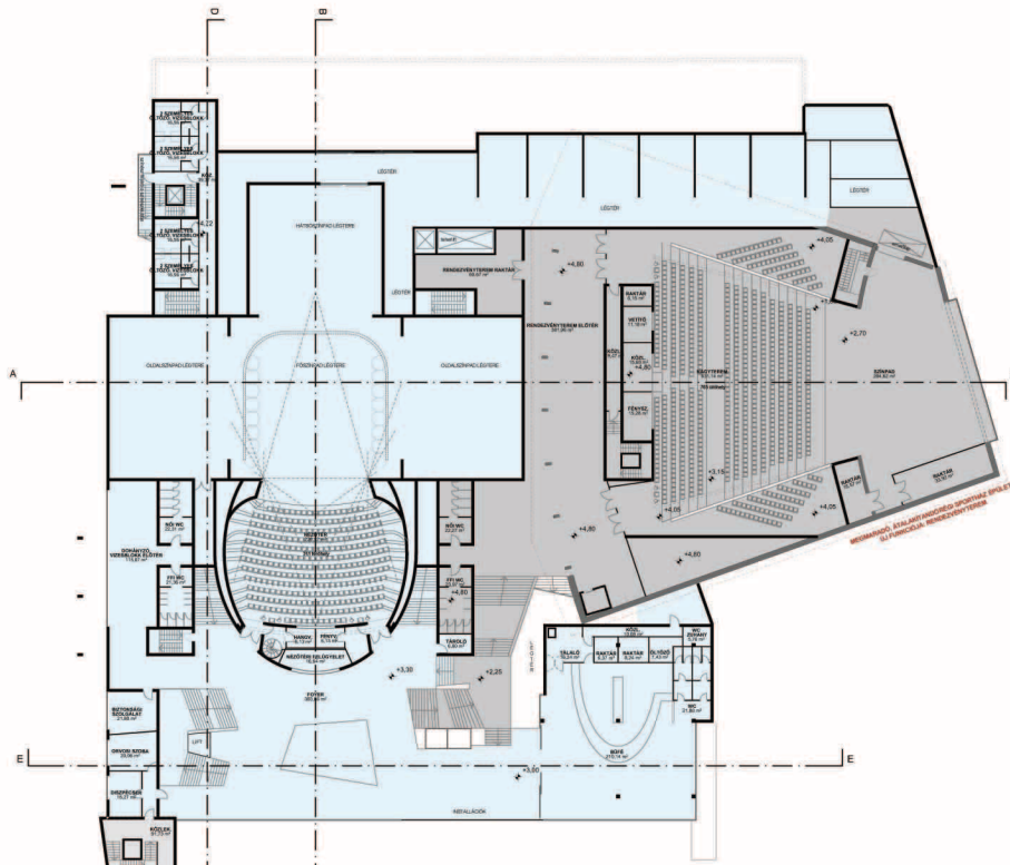
1. szint alaprajza nézőtér, büfé, konferenciaterem, tv stúdió irodái
