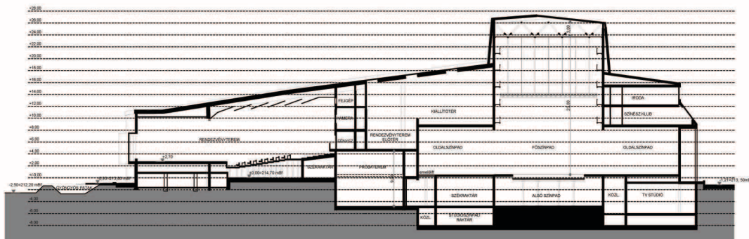
a-a metszet
