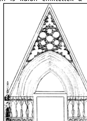
A Mária templom kapujának rekonstrukciós képe az előkerült kövek alapján (Bertalan, 1995)
