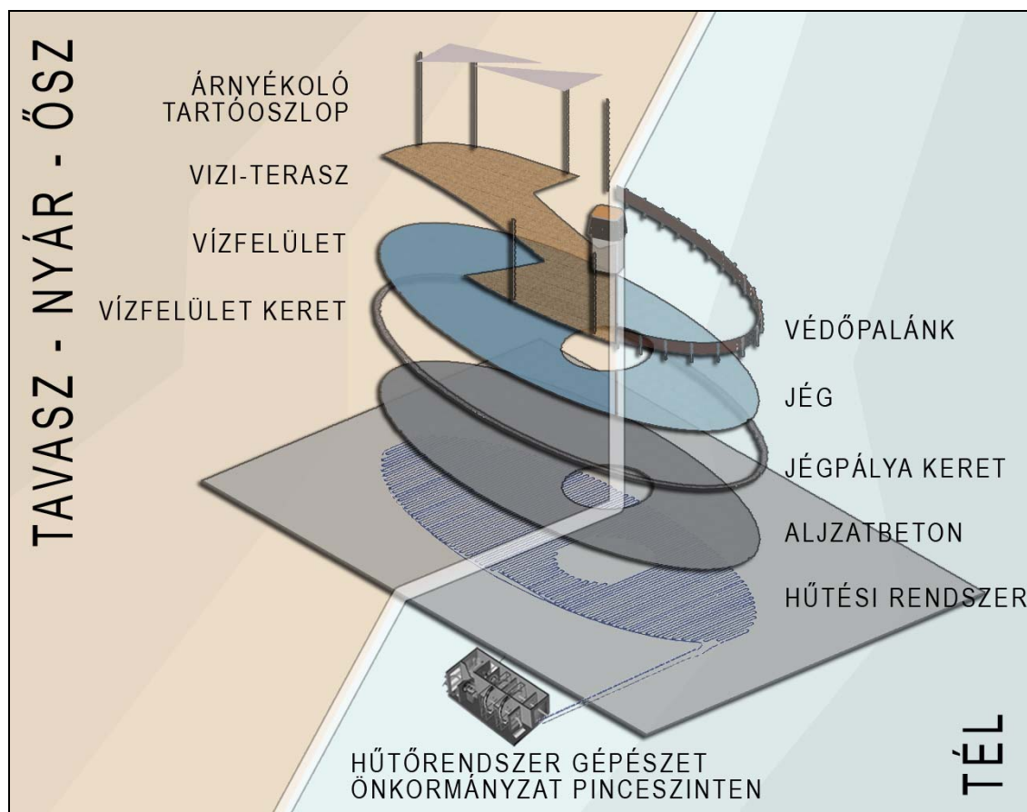
A medence / korcsolyapálya elvi sémája
