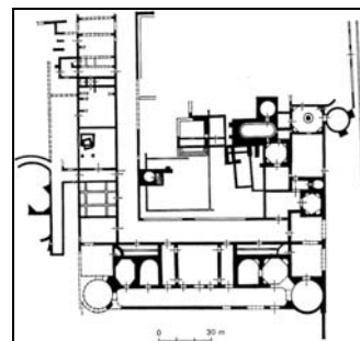
A helytartói palota alaprajza (Szilágyi, 1956)
