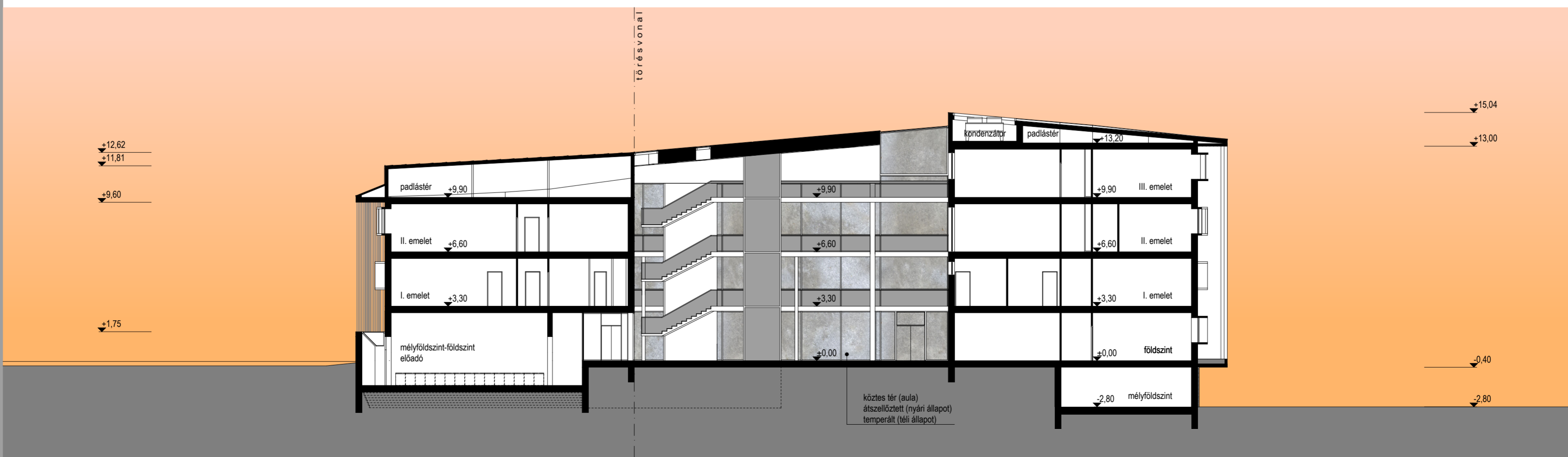
D-D METSZET M 1:200
