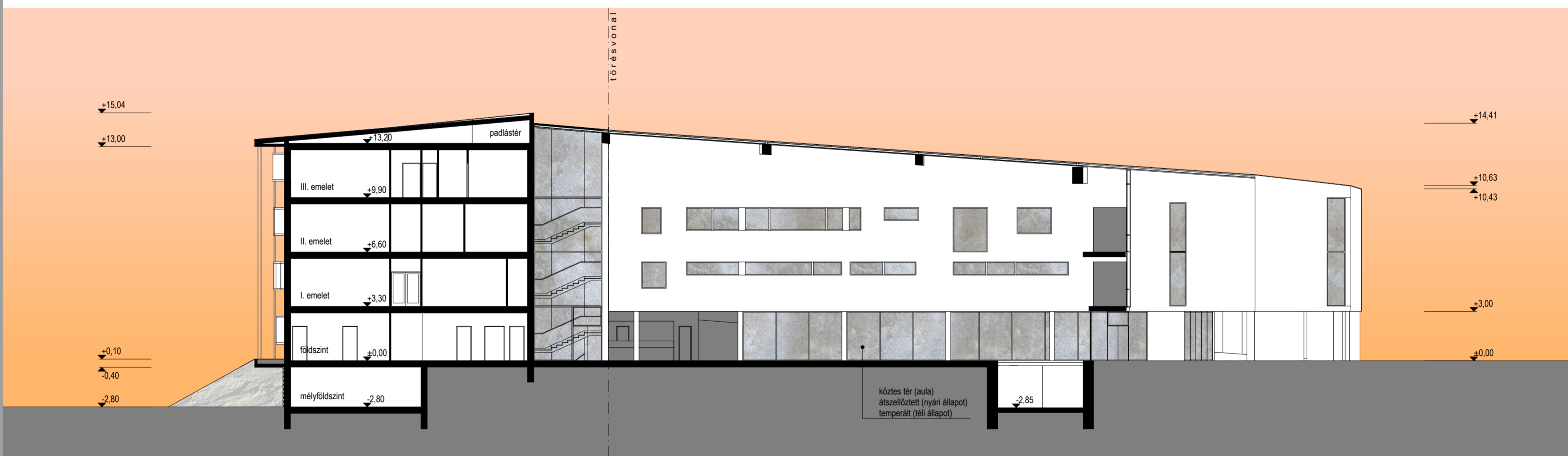
C-C METSZET M 1:200
