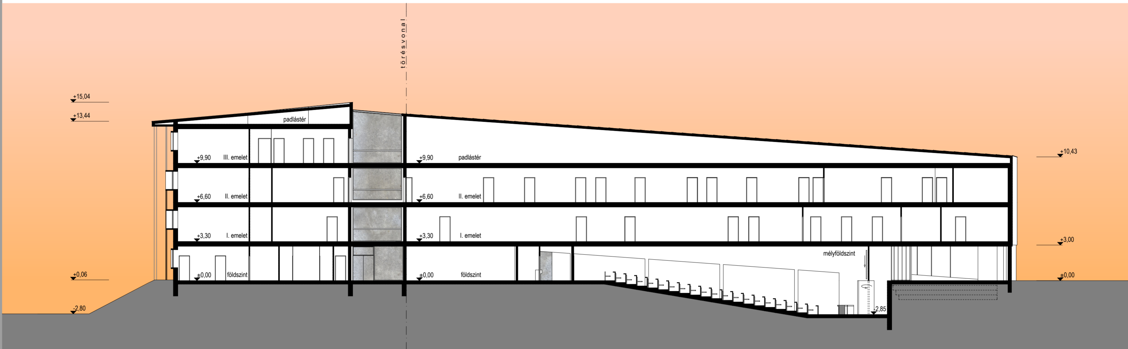
B-B METSZET M 1:200
