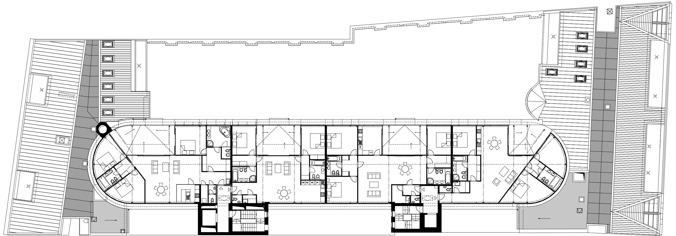
UDVARI TETŐTÉR ALAPRAJZ
