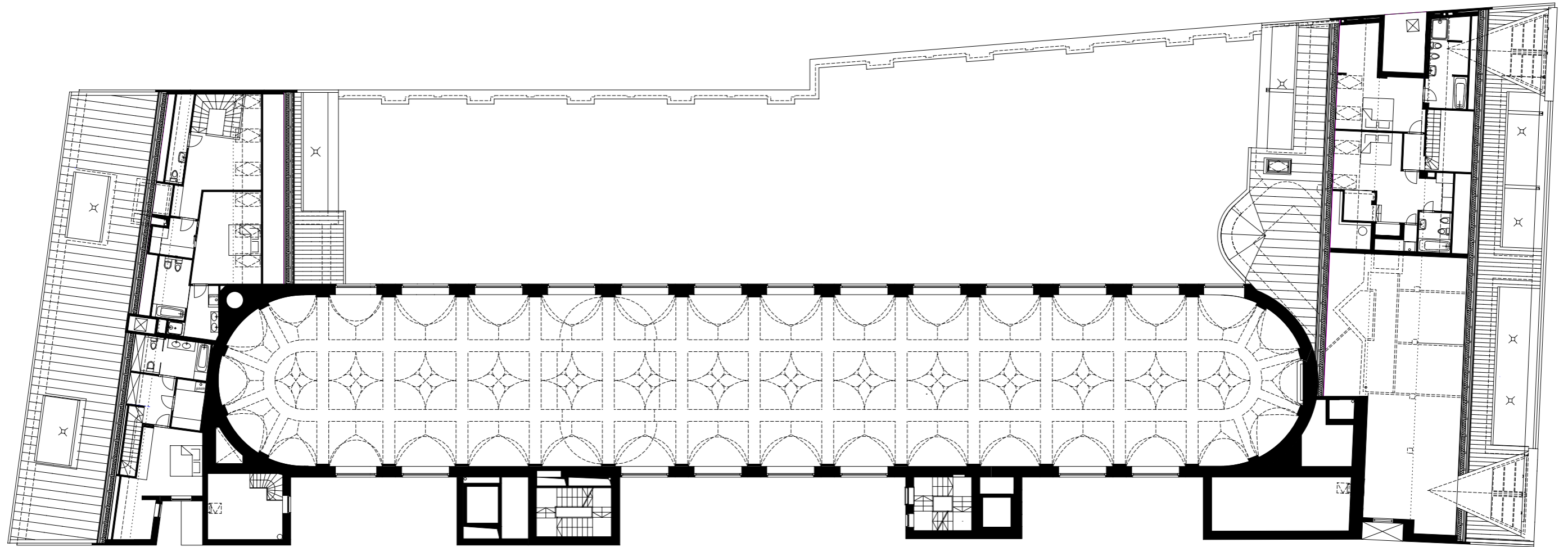
UTCAI TETŐTÉR GALÉRIA ALAPRAJZ
