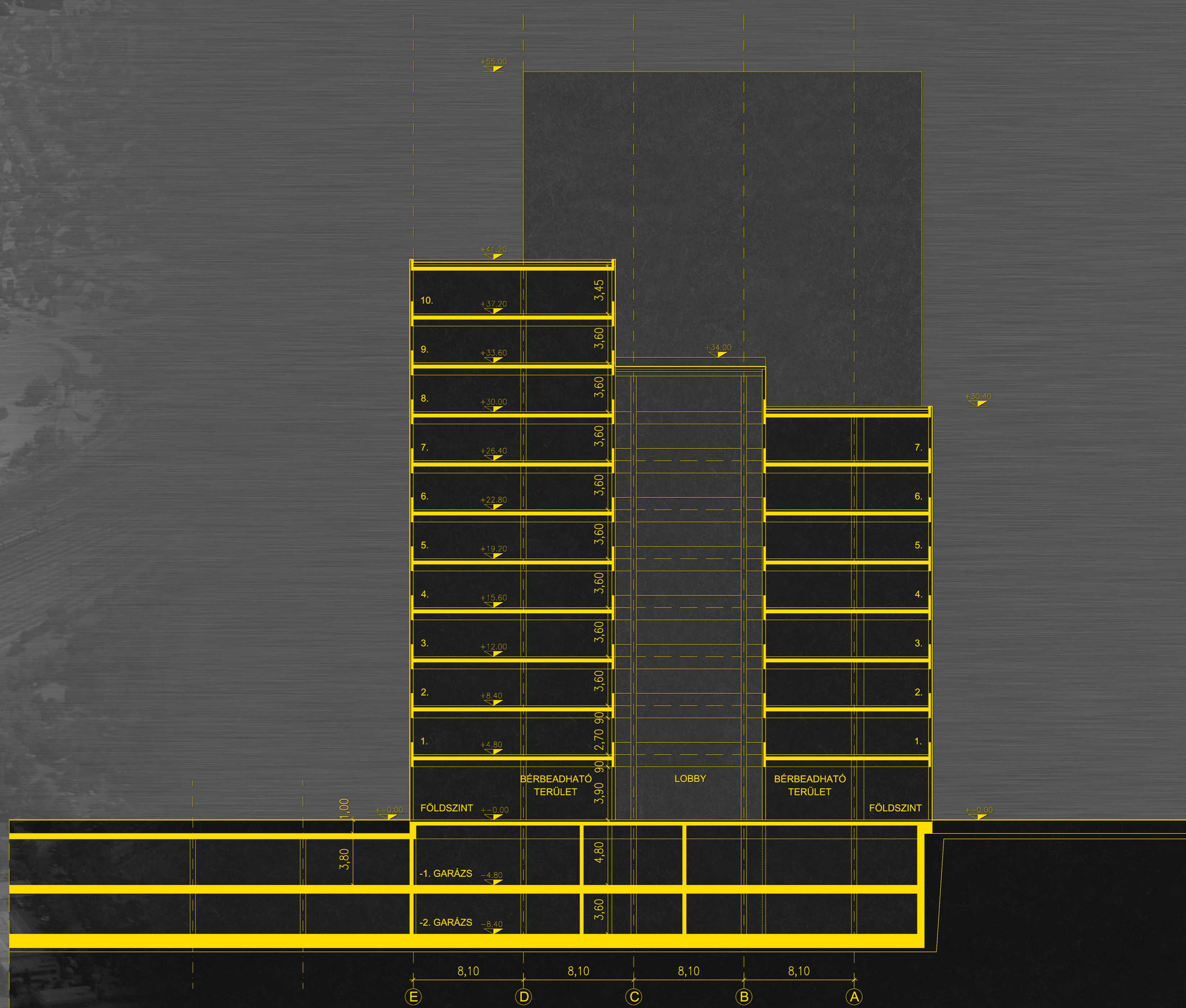
keresztmetszet
