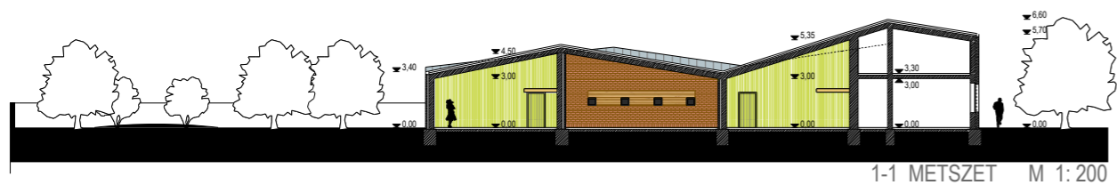
1-1 METSZET M 1:200
