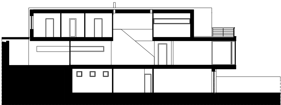
metszet
