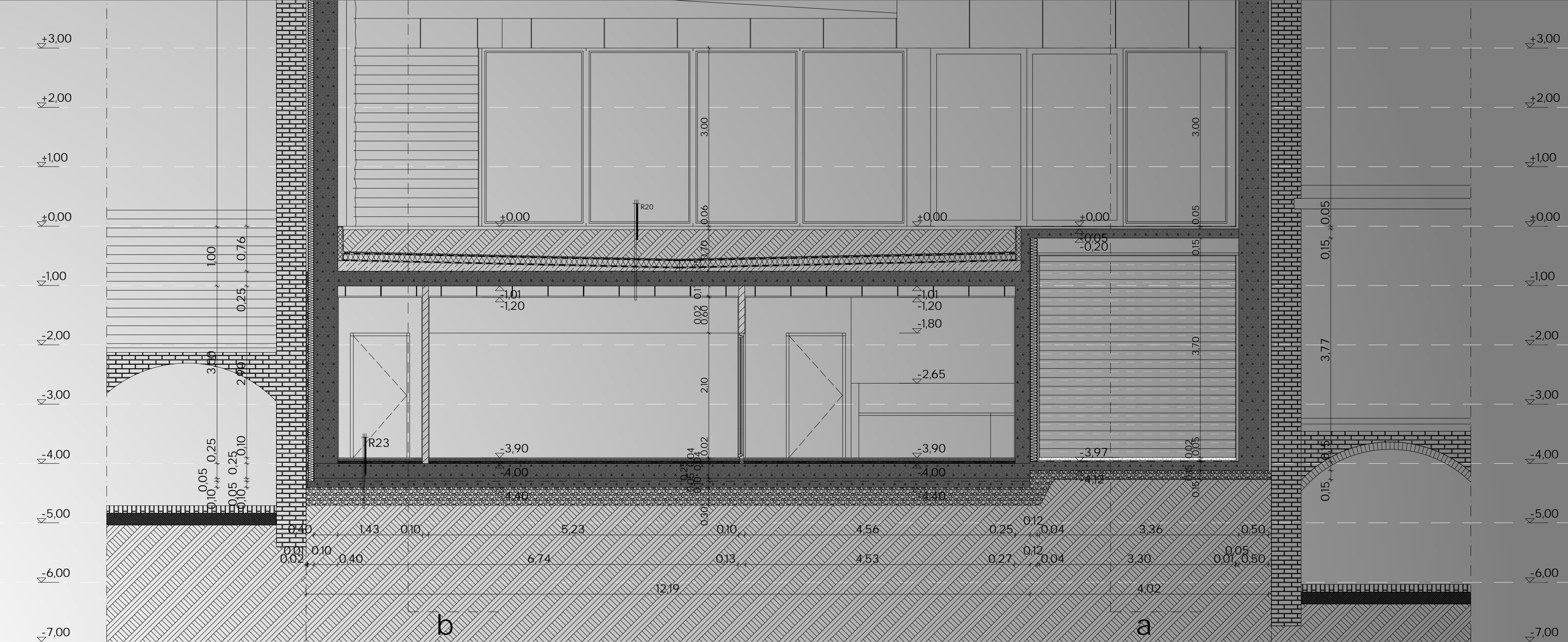
c-c rész metszet
