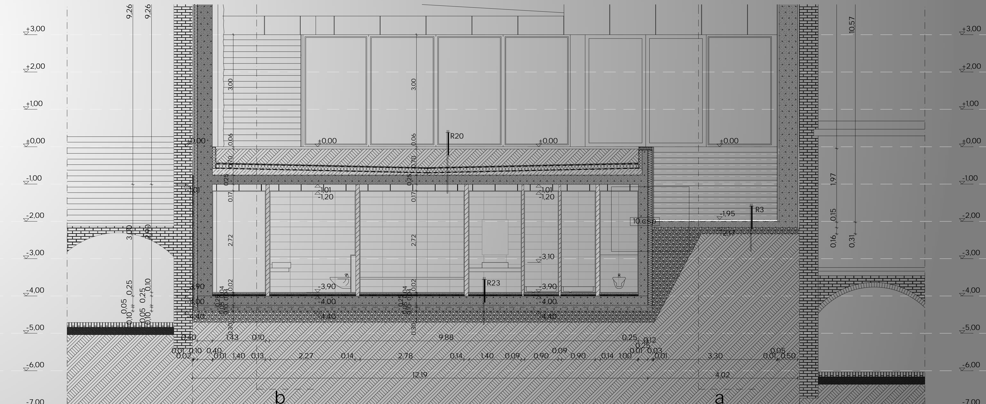
d-d rész metszet
