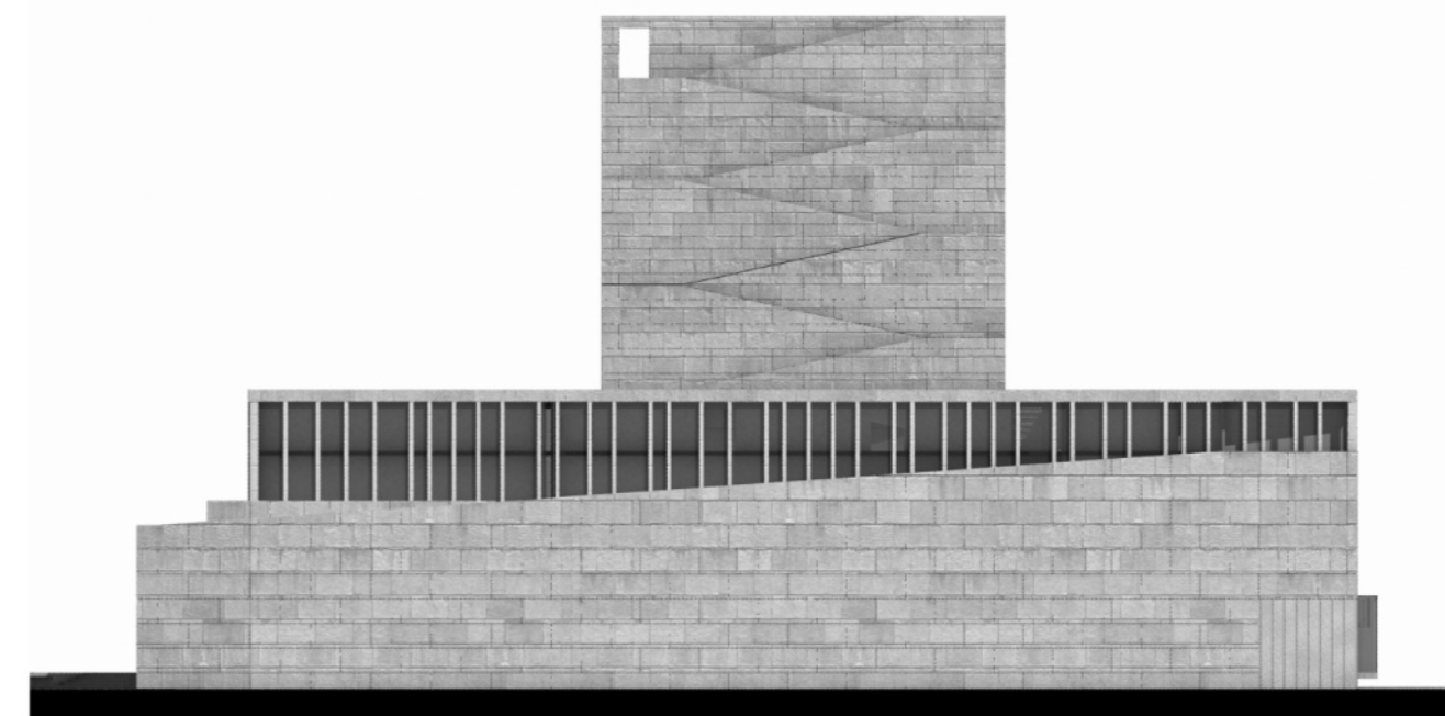
18-AS HONVÉD UTCA FELŐLI HOMLOKZAT
