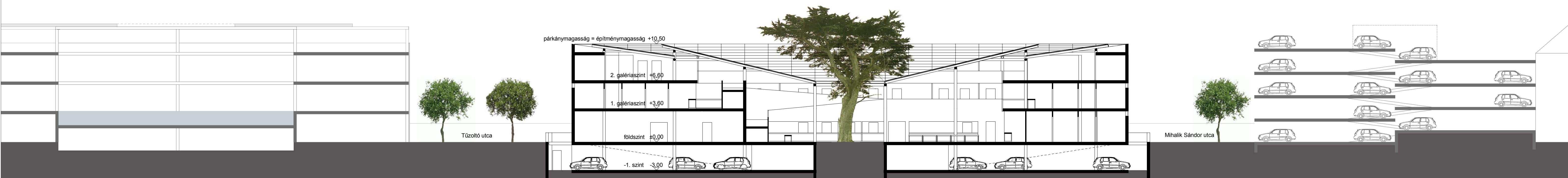
b-b metszet (a távlati környezetbe illesztve) m=1:200
