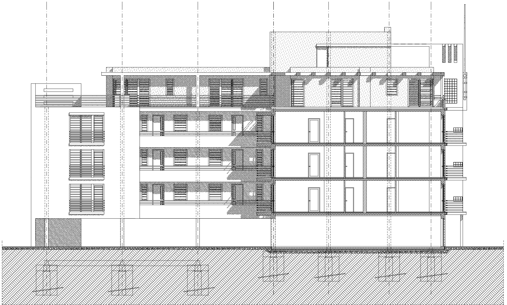
ÉSZAKI HOMLOKZAT
