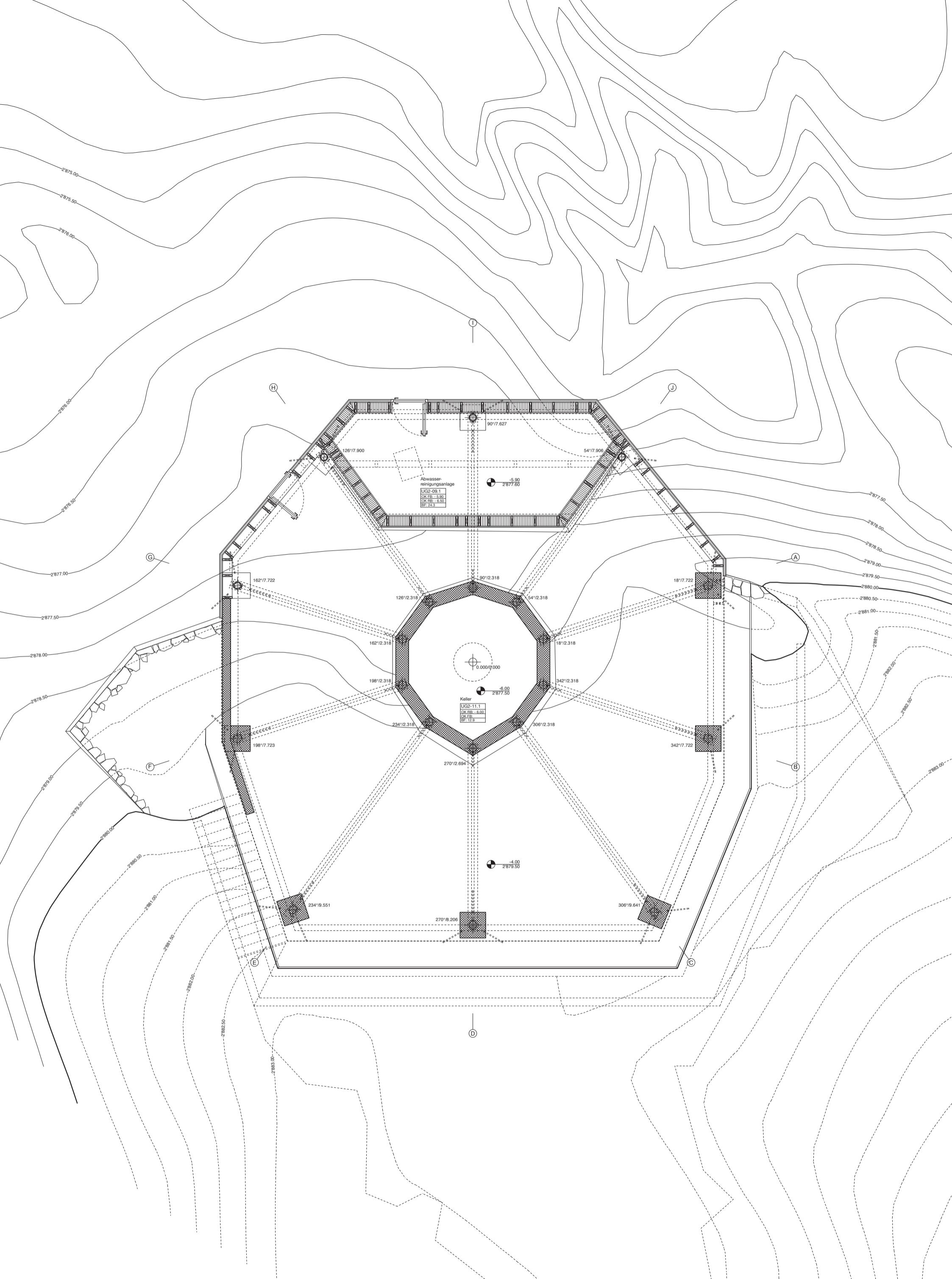
Neue Monte-Rosa-Hütte SAC, Grundriss 2. Untergeschoss, Mst. 1:100 © ETH-Studio Monte Rosa, Prof. Andrea Deplazes, ETH Zürich
