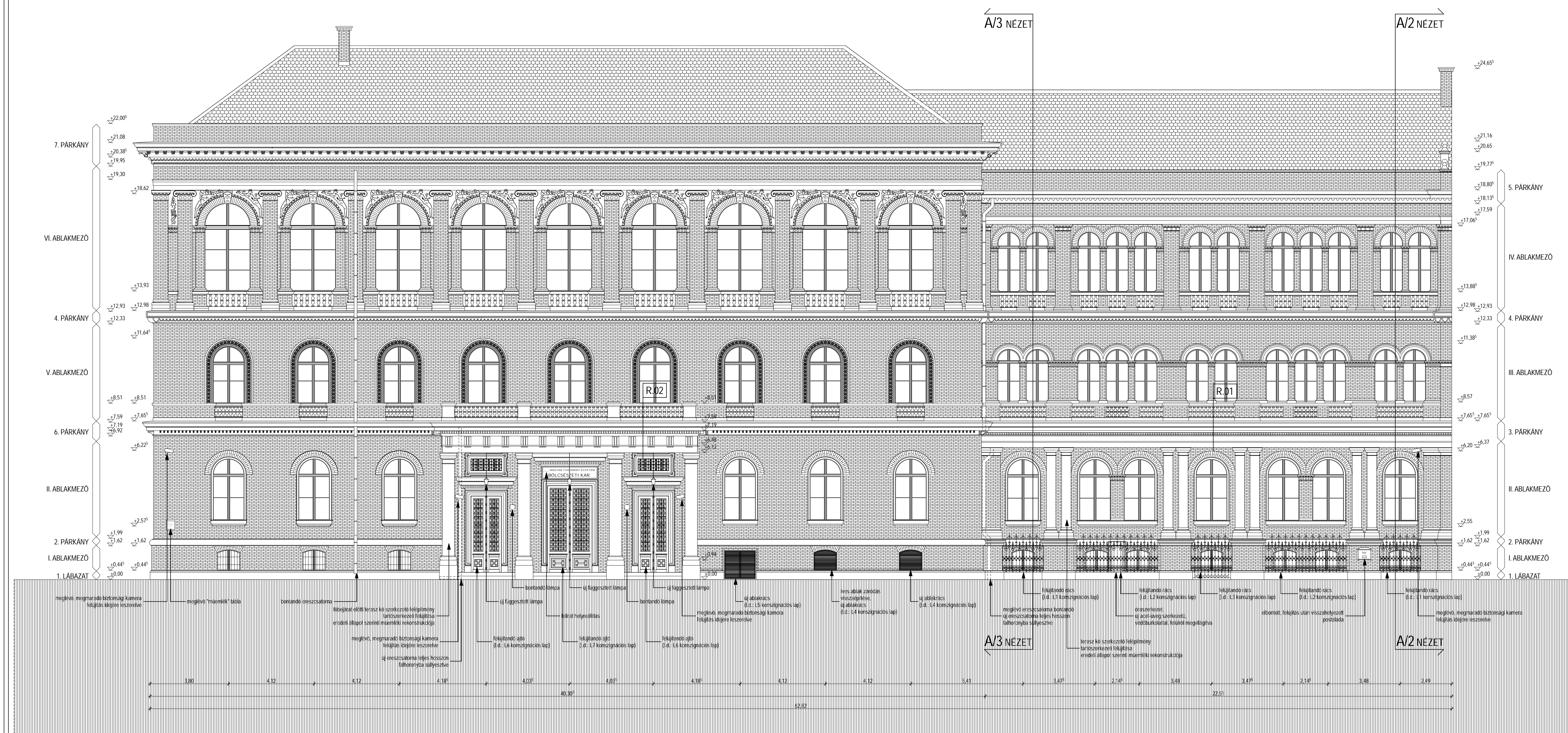
A/1 HOMLOKZATI NÉZET
