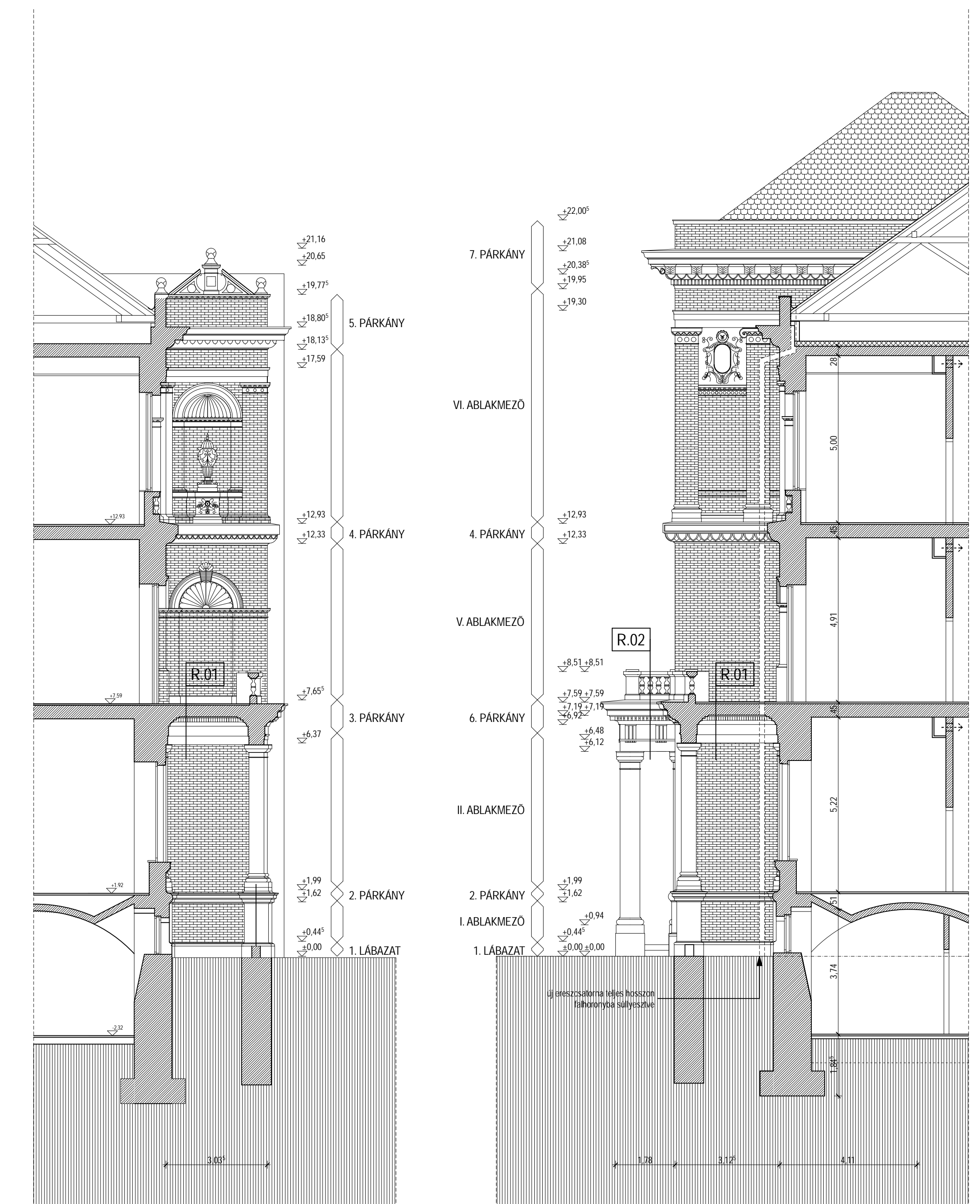
A/2 HOMLOKZATI NÉZET
