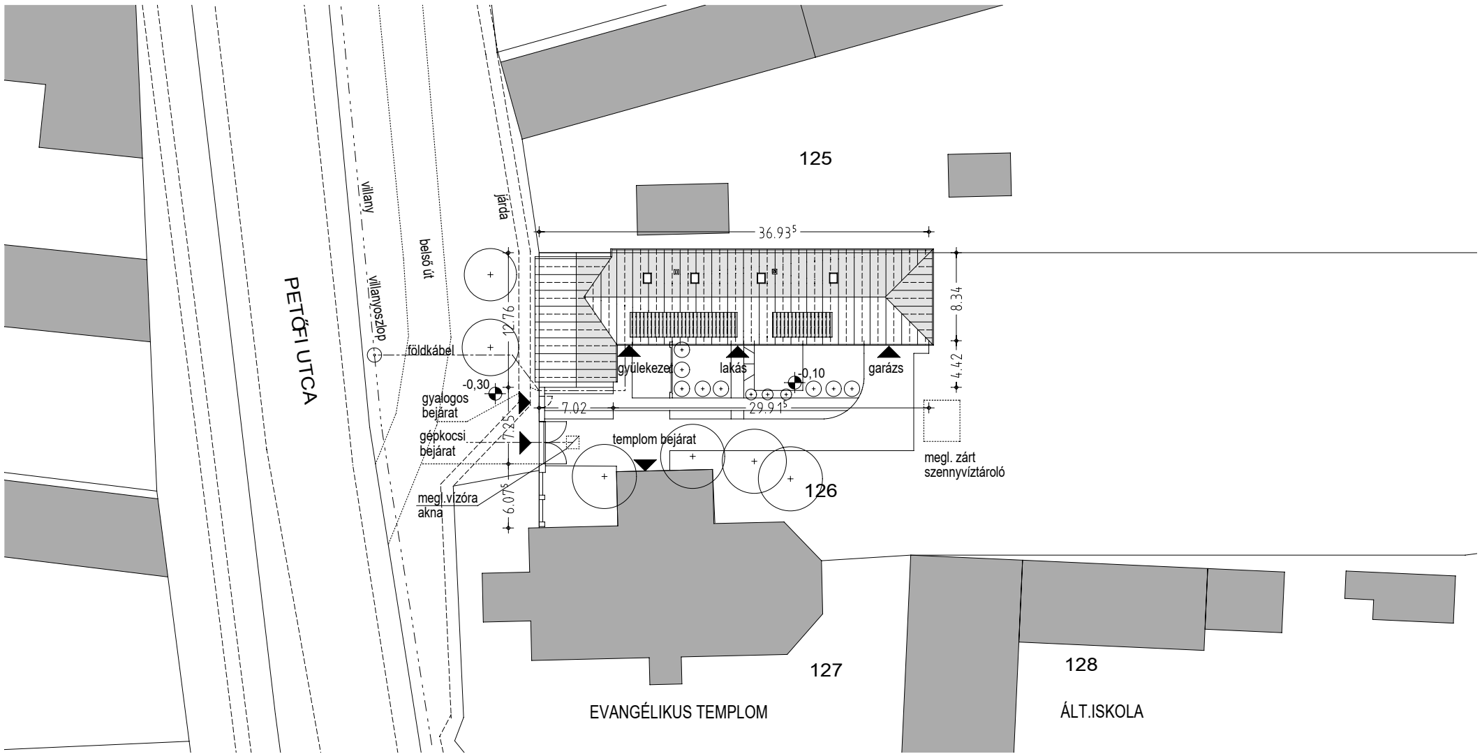
SÁRSZENTLŐRINC - EVANGÉLIKUS PARÓKIA HELYSZÍNRAJZ M = 1:500
