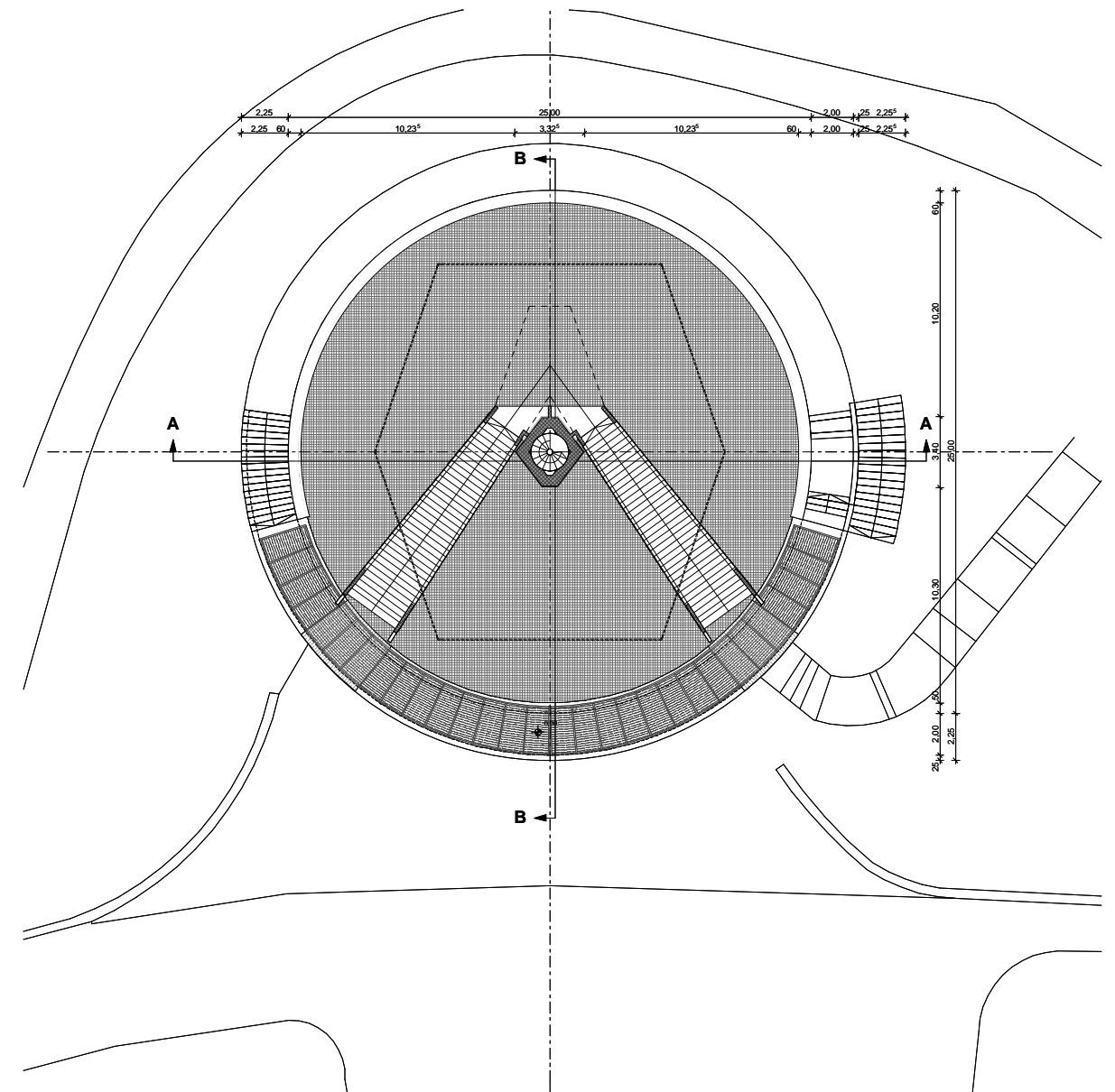
FOLDSZINT ALAPRAJZ
