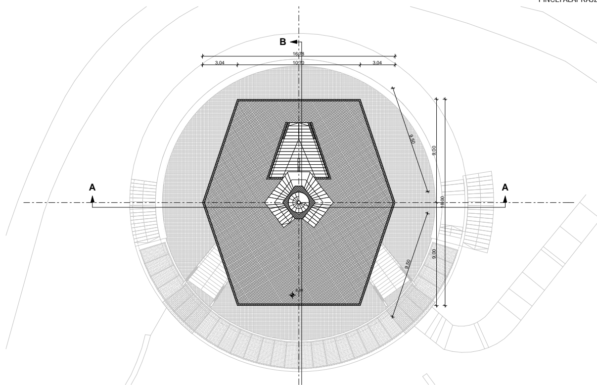
1.EMELET ALAPRAJZ
