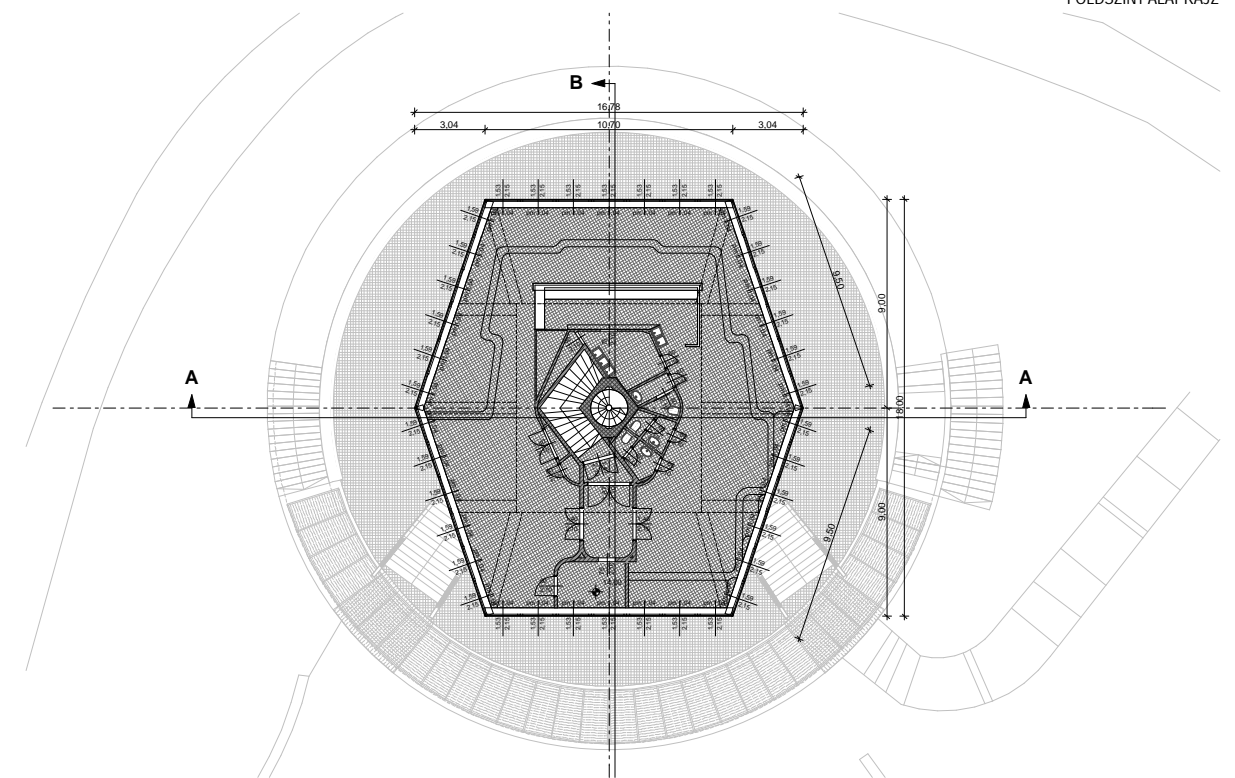
2.EMELET ALAPRAJZ
