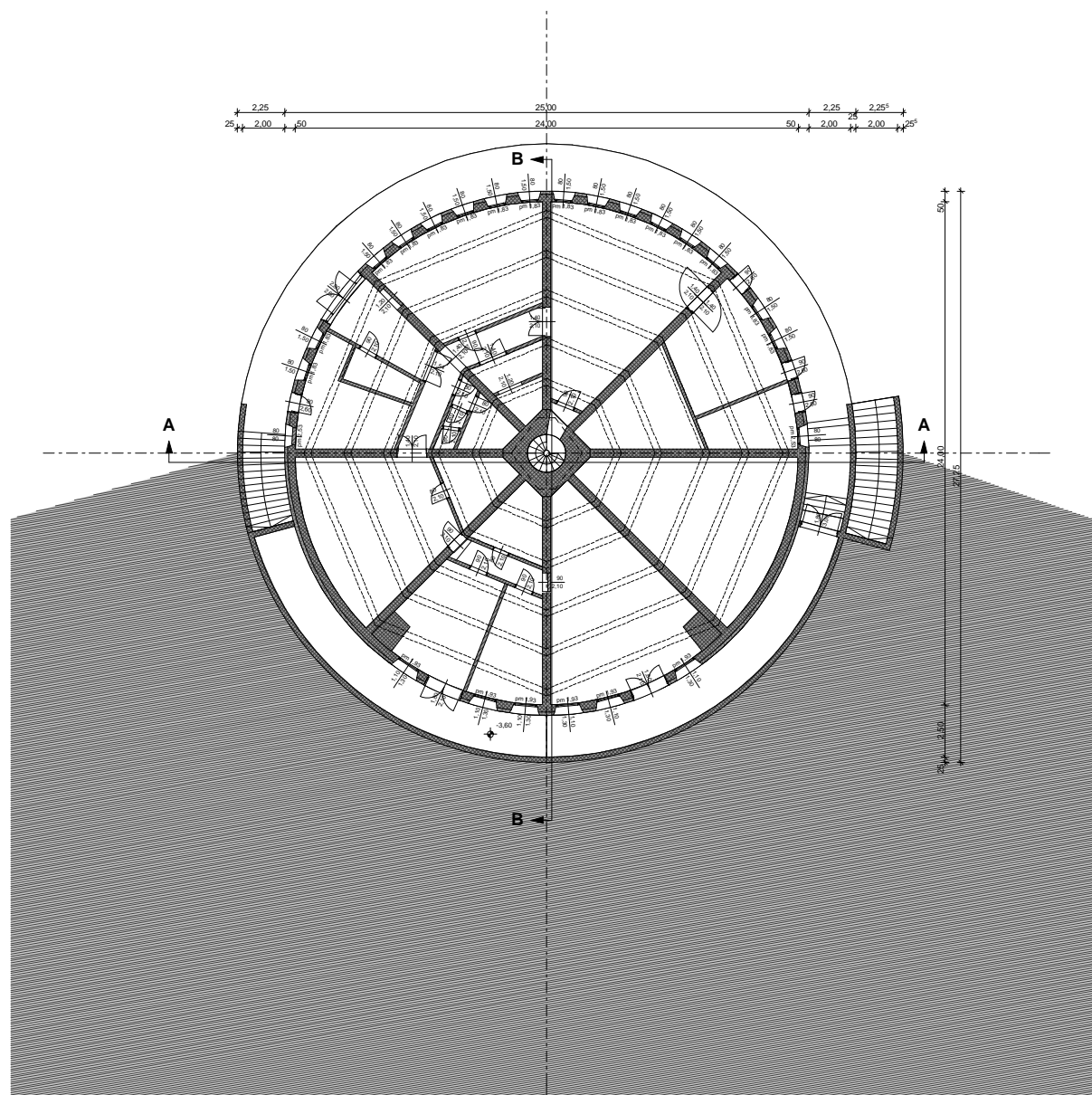
PINCEI ALAPRAJZ
