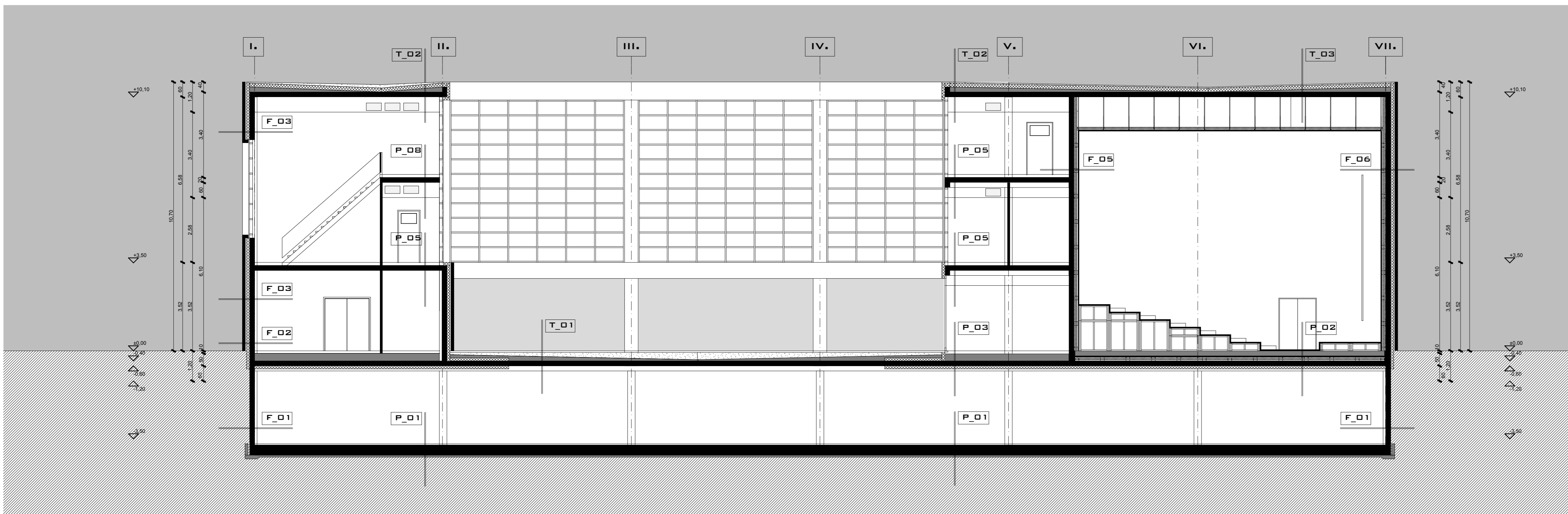
B-B METSZET - UTCÁVAL PÁRHUZAMOS FŐMETSZET - M=1:100
