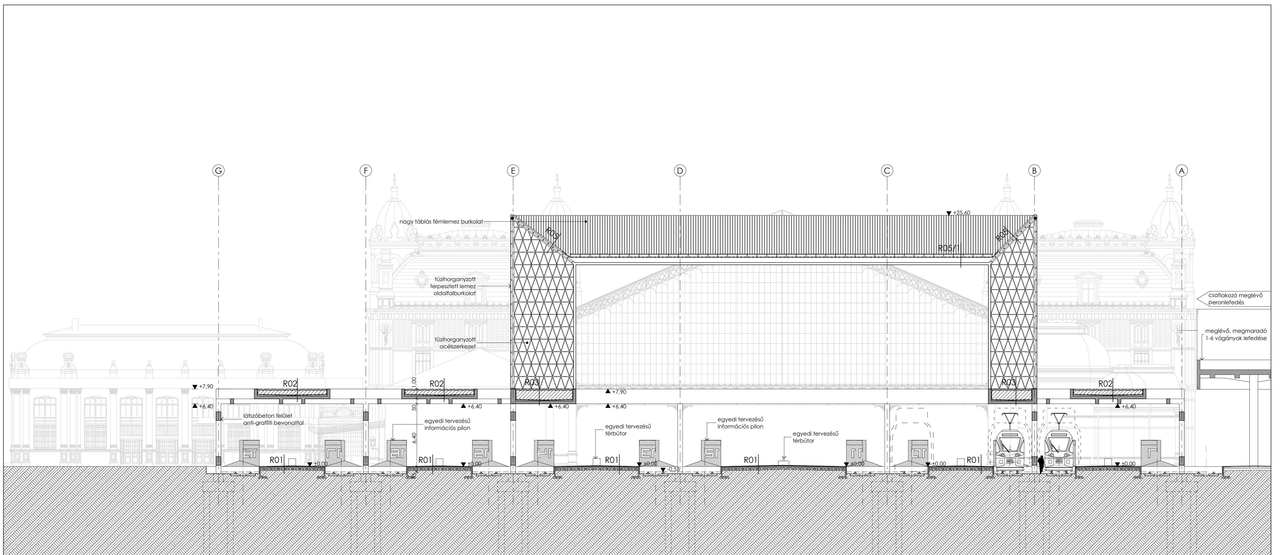
4-4 KERESZTMETSZET
