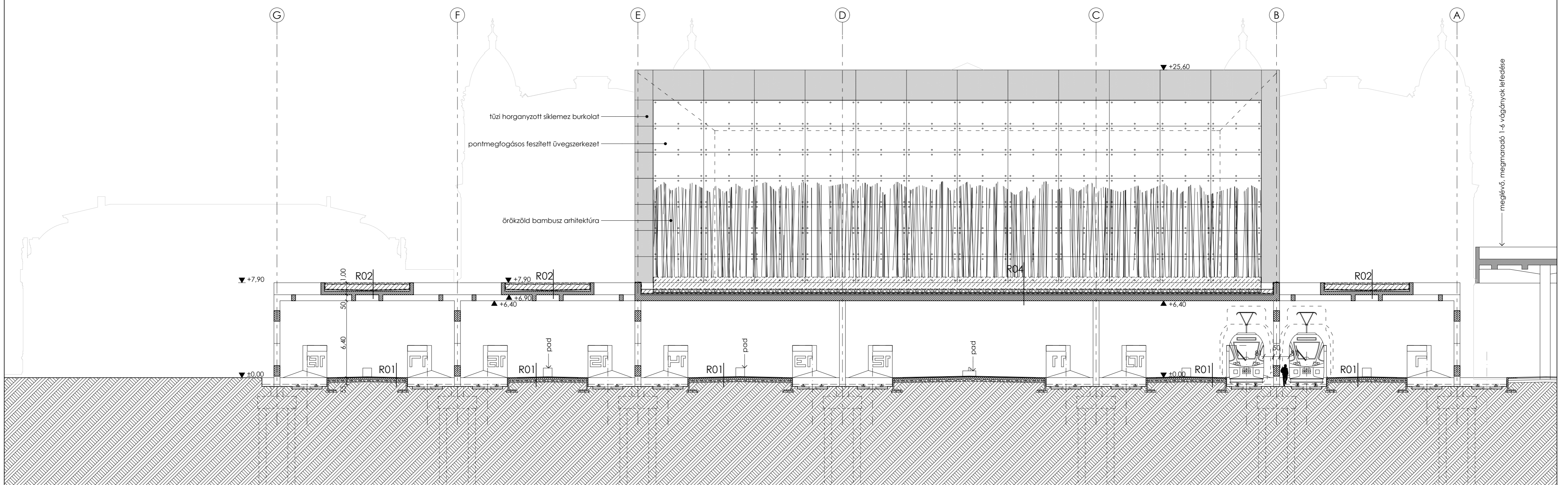
5-5 KERESZTMETSZET
