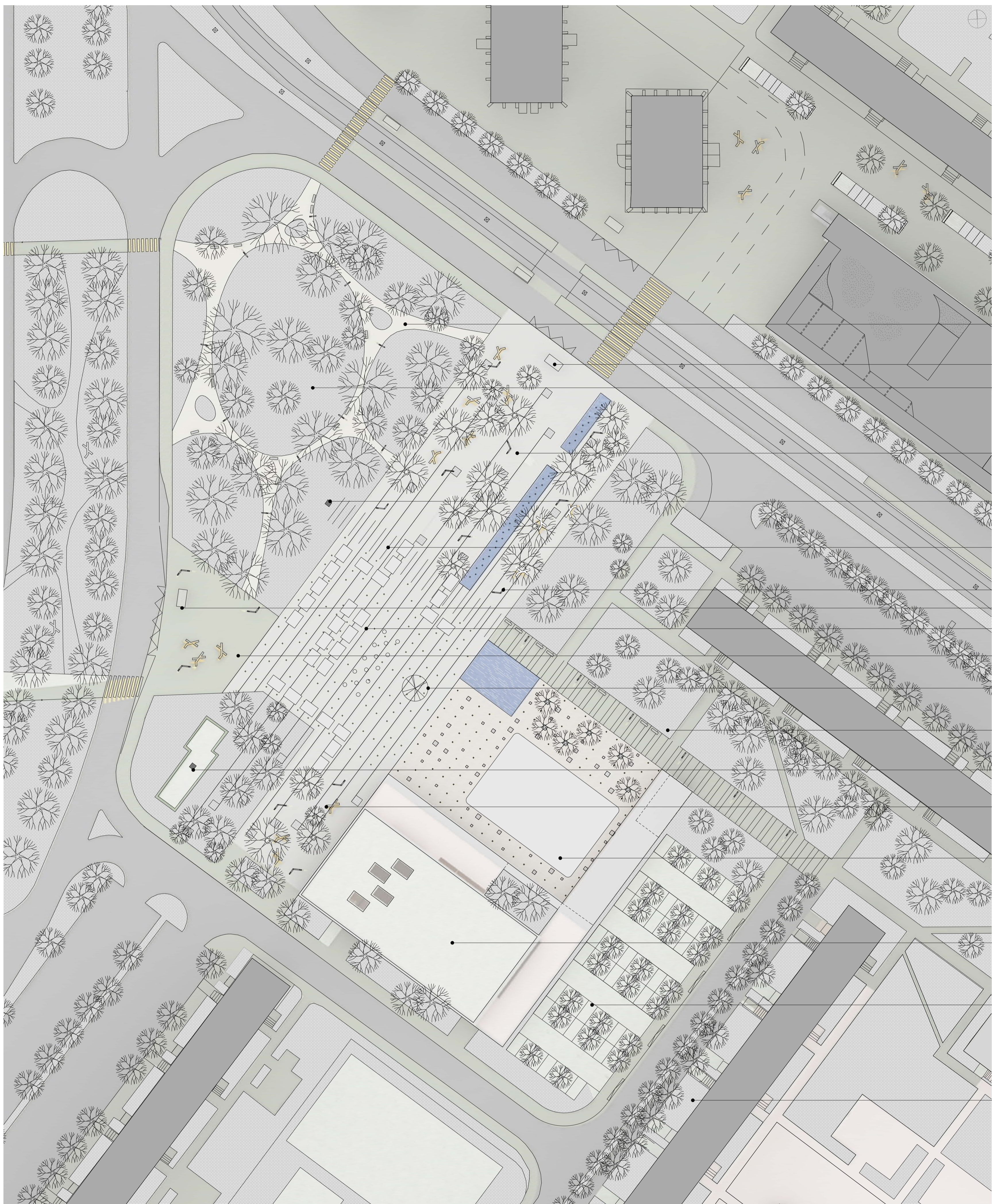
TÉLI HELYSZÍNRAJZ M 1:500
