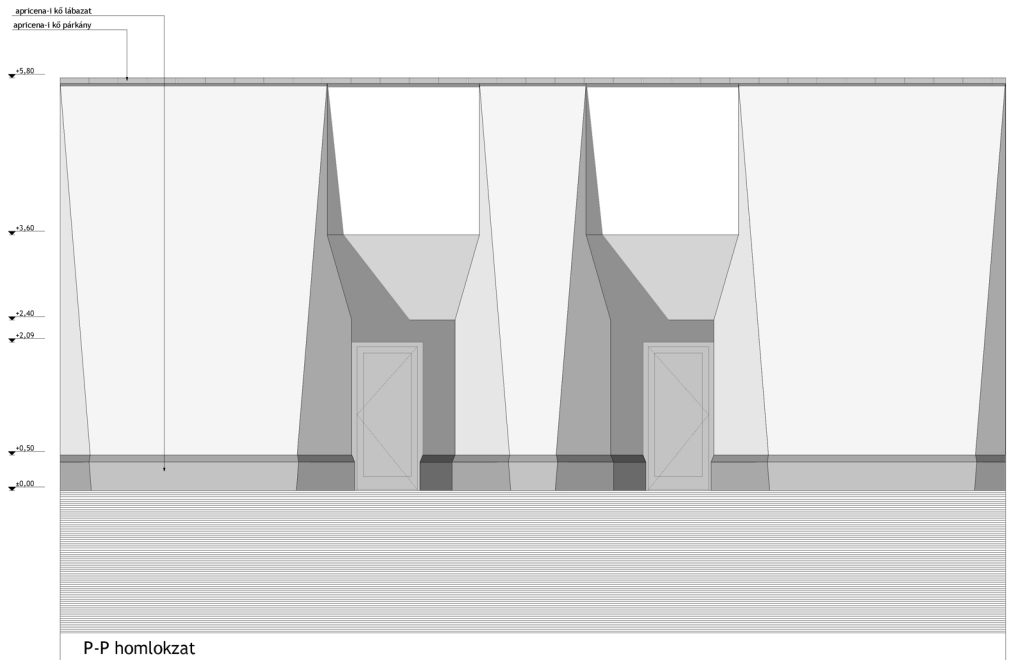
P-P homlokzat
