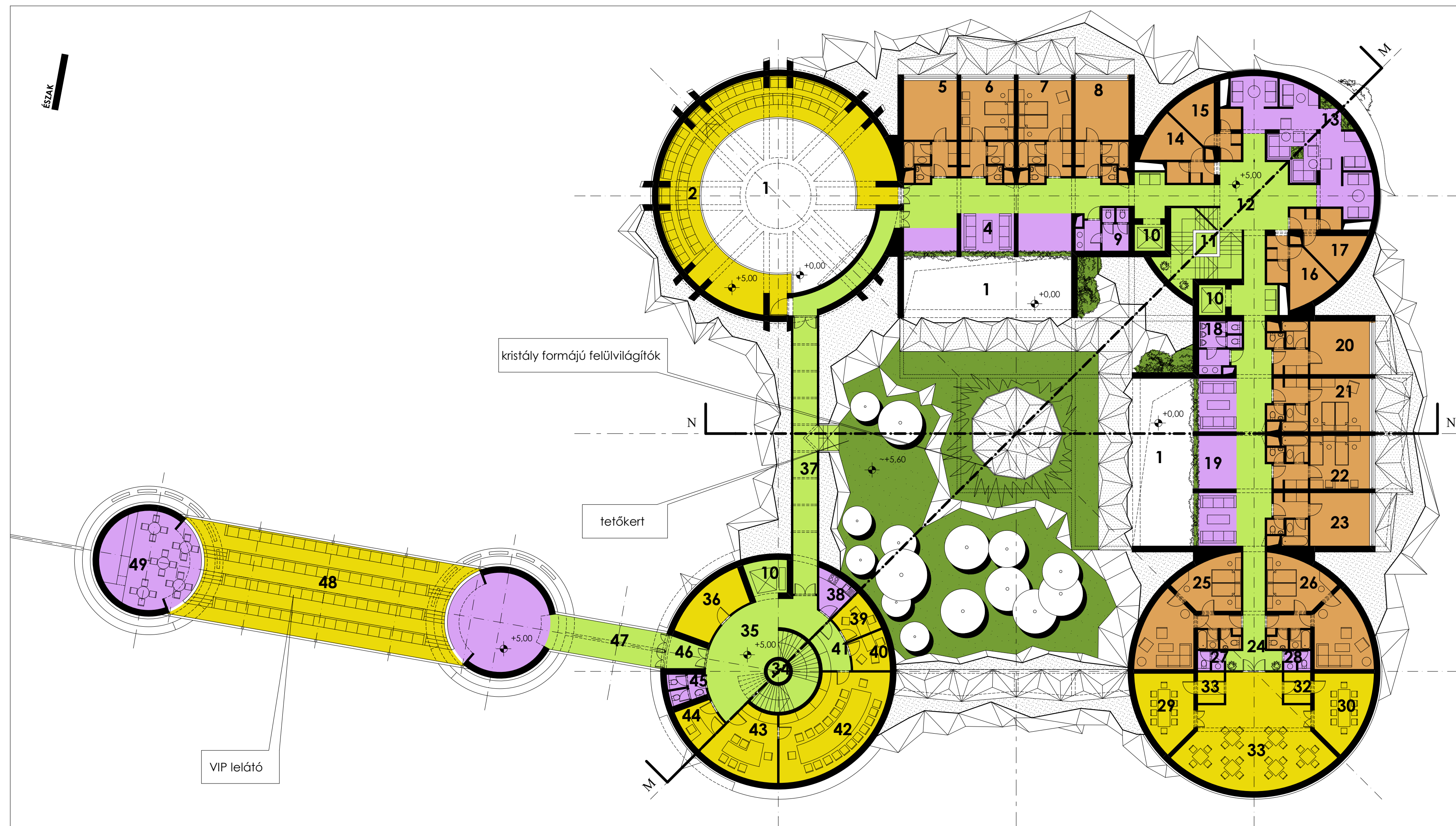
ELSŐ EMELETI ALAPRAJZ lépték 1:200
