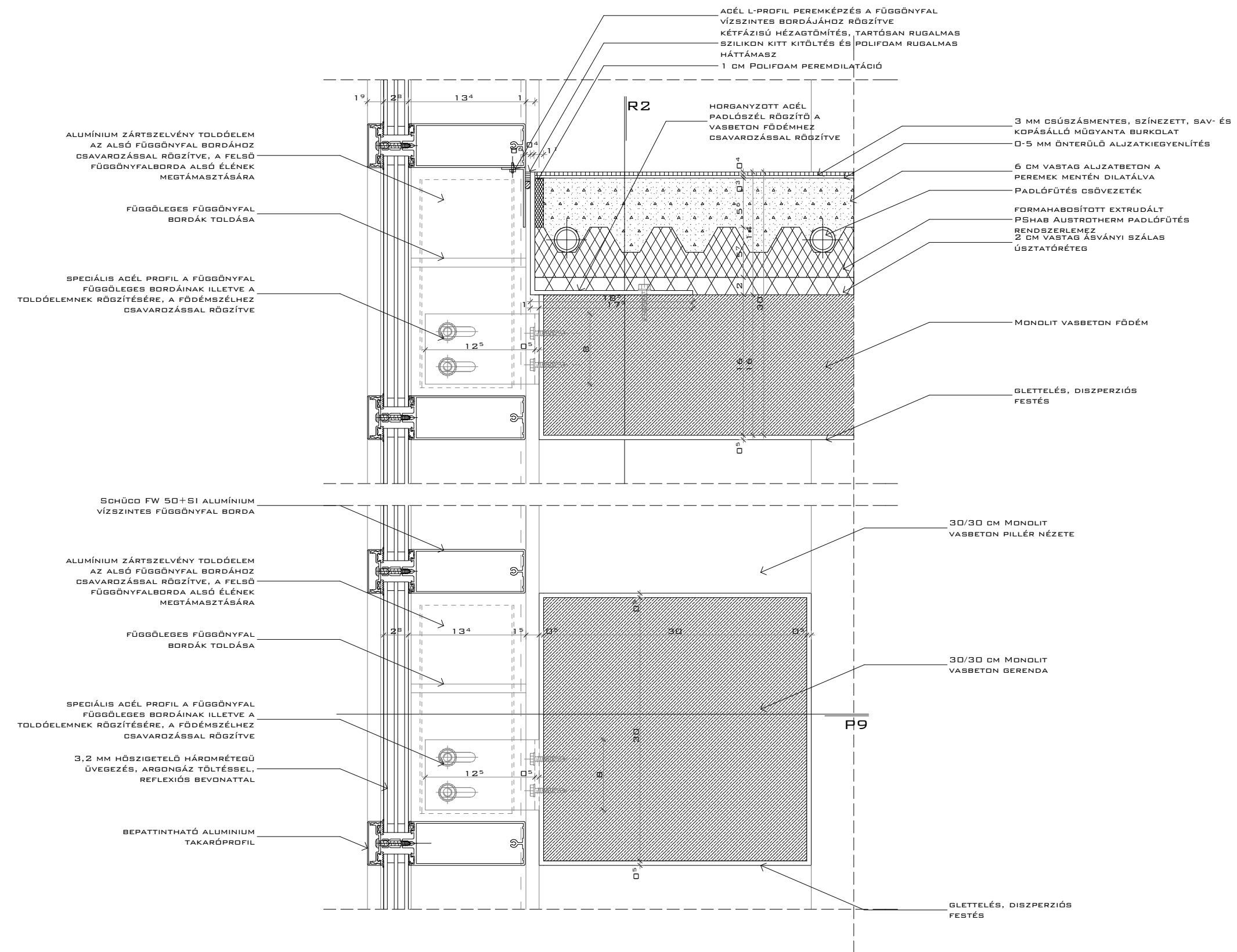
4-5. CSOMÓPONT FÜGGÖNYFAL ÉS FÖDÉMSZÉL/GERENDA CSATLAKOZÁSA
