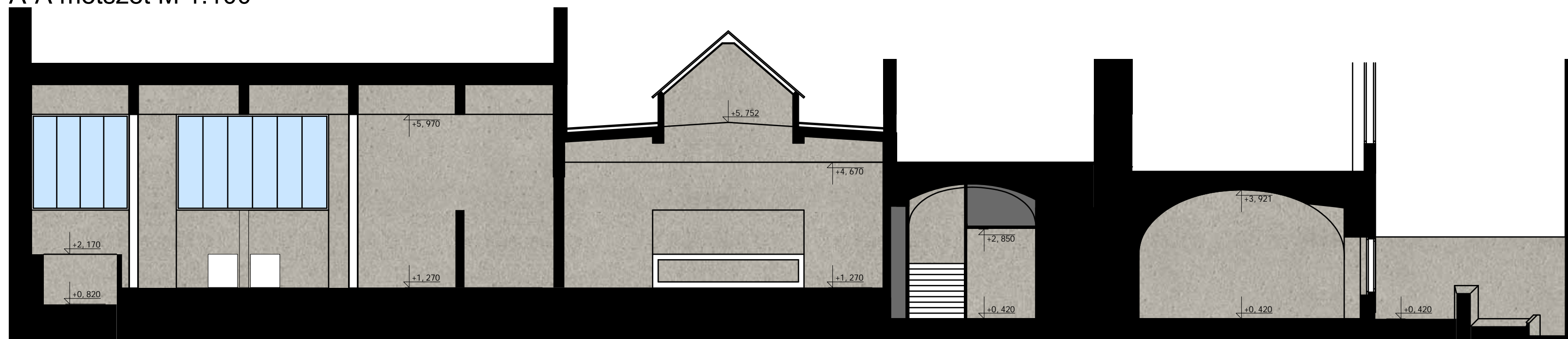
A-A metszet M 1:100
