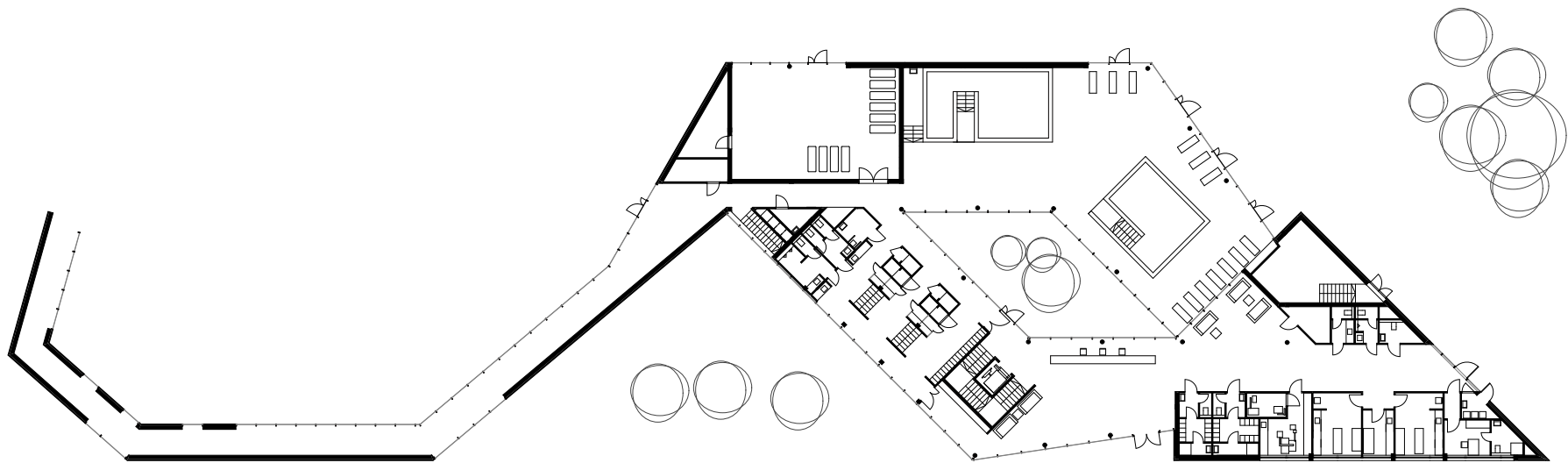
Pápa, Gyógy- és termálfürdő, Gyógyászat földszinti alaprajz
