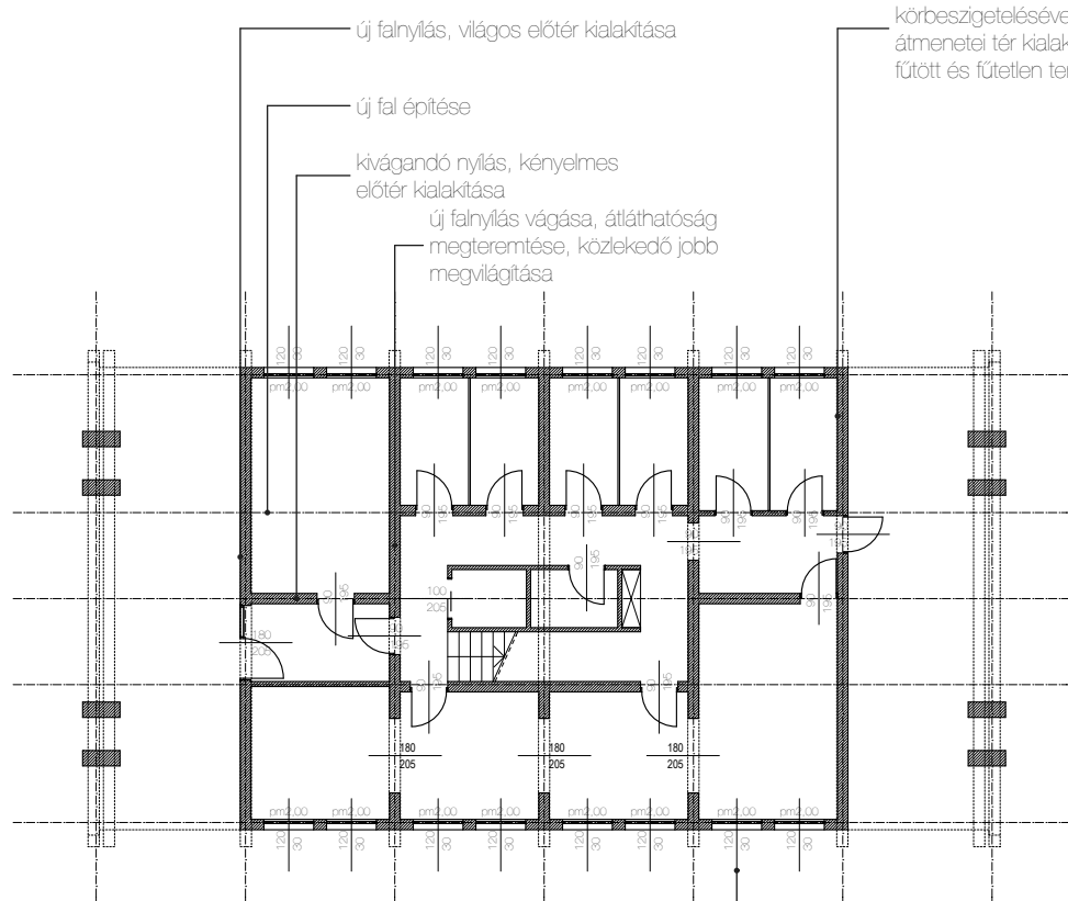
termikus burk az épület körül
