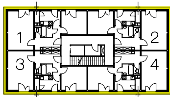
termikus burk az épület körül
