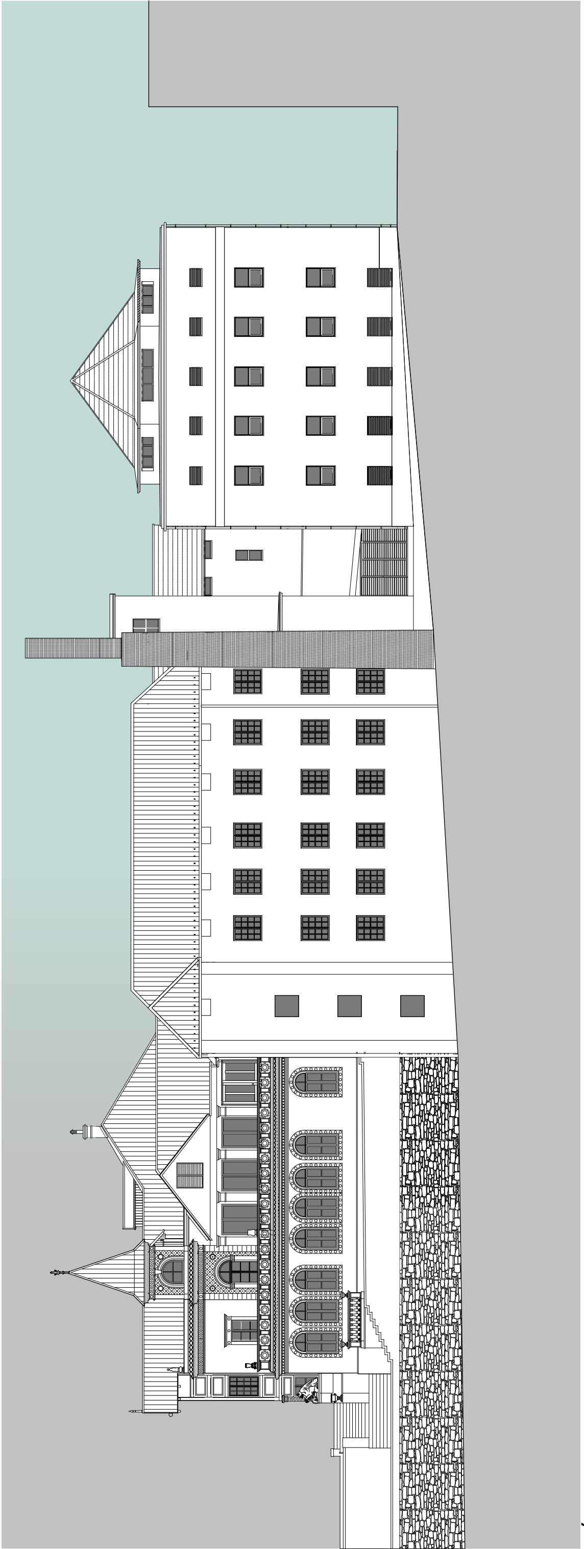
DÉLI HOMLOKZAT
