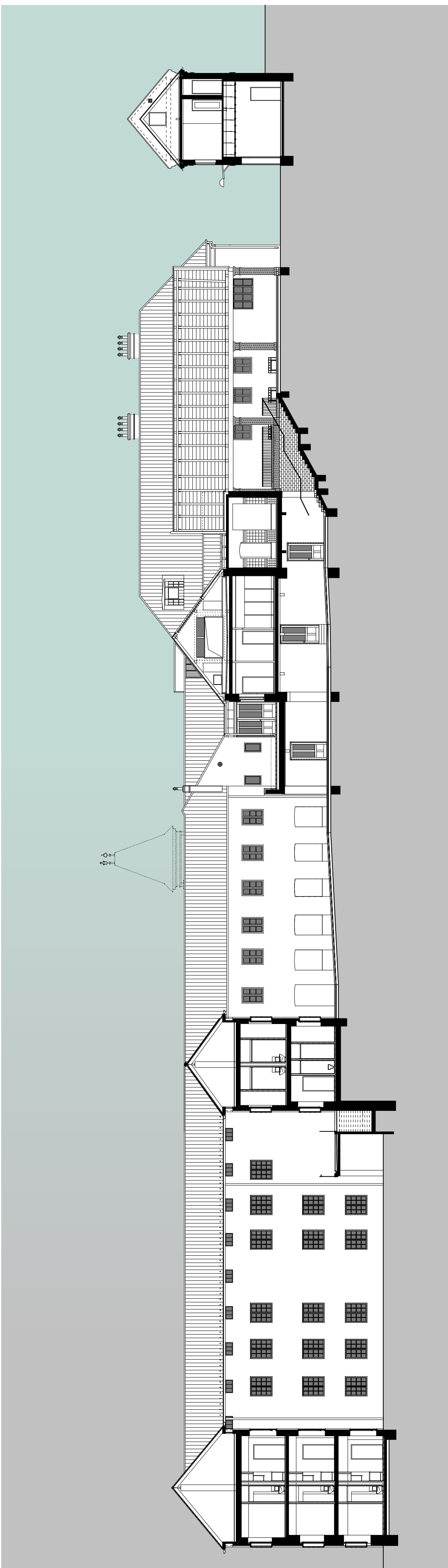
HOSSZMETSZET
