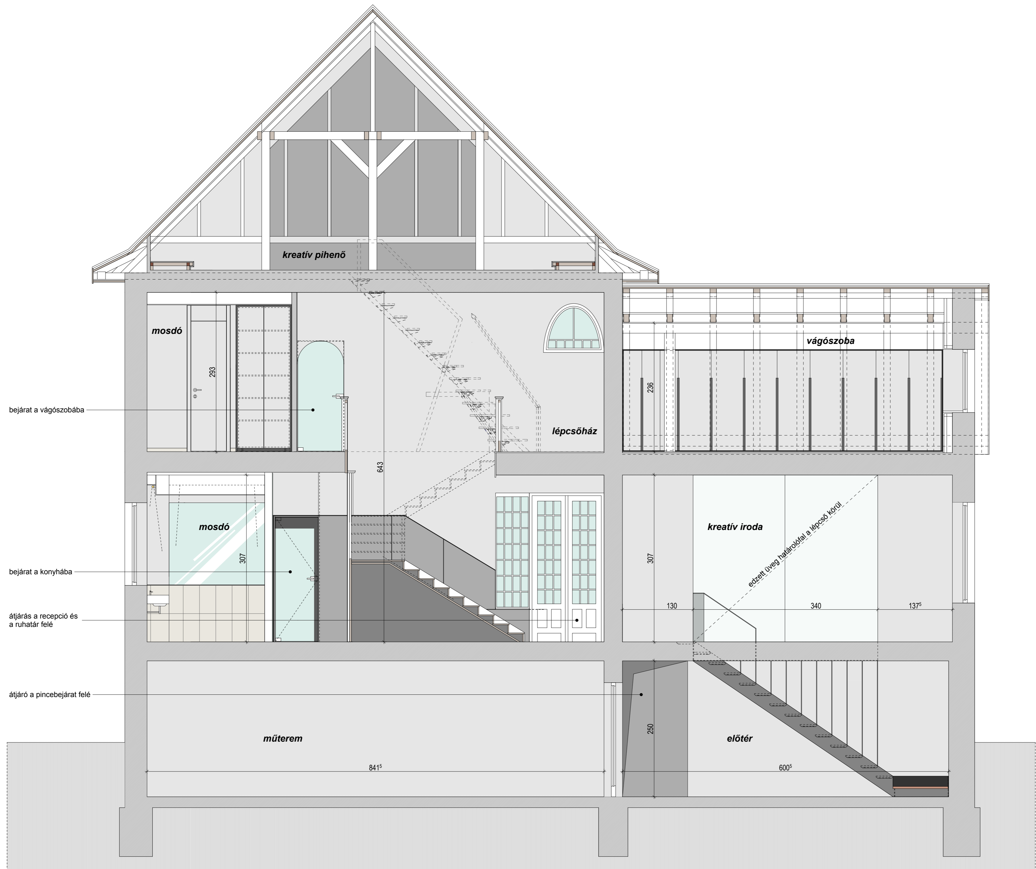
metszet, nézet a lépcsőházban a közlekedő felé
