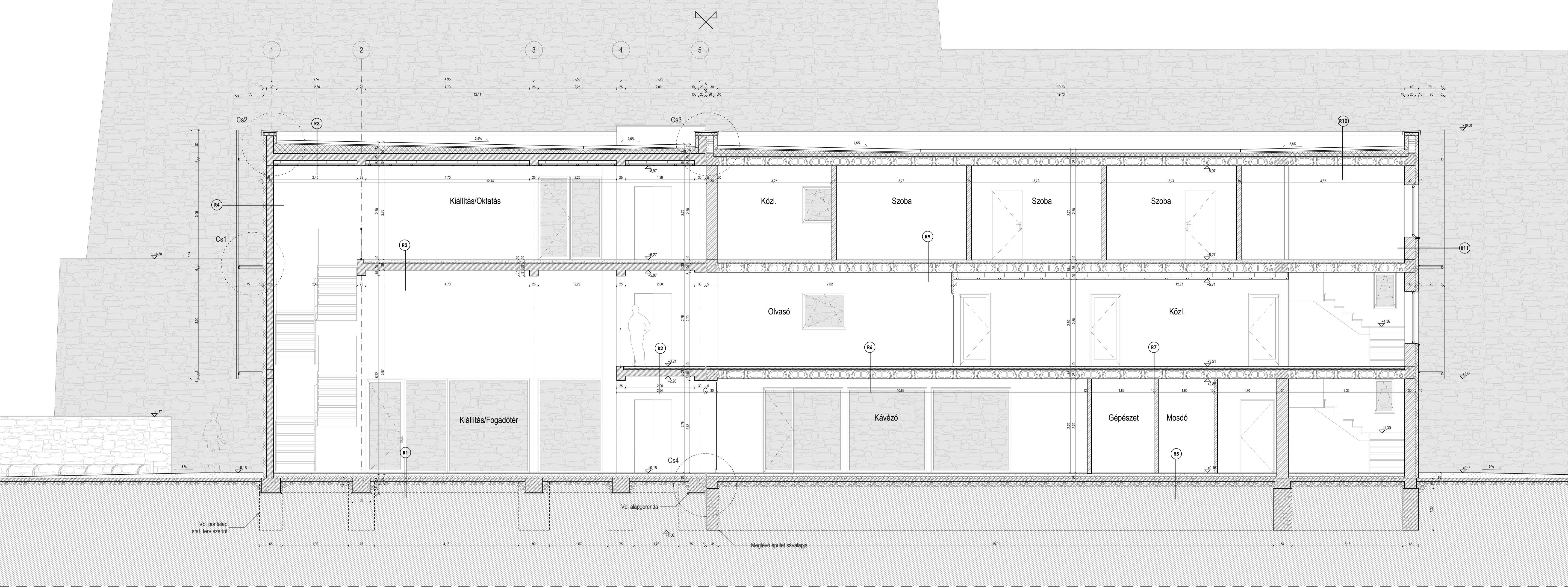
A-A METSZET M=1:50
