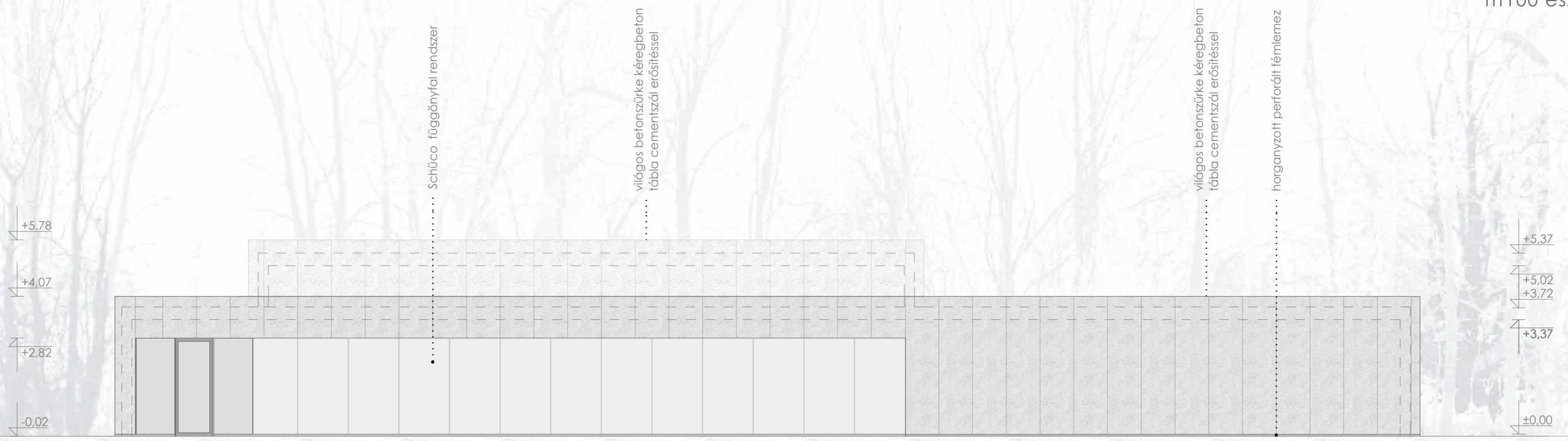
m100 északi homlokzat
