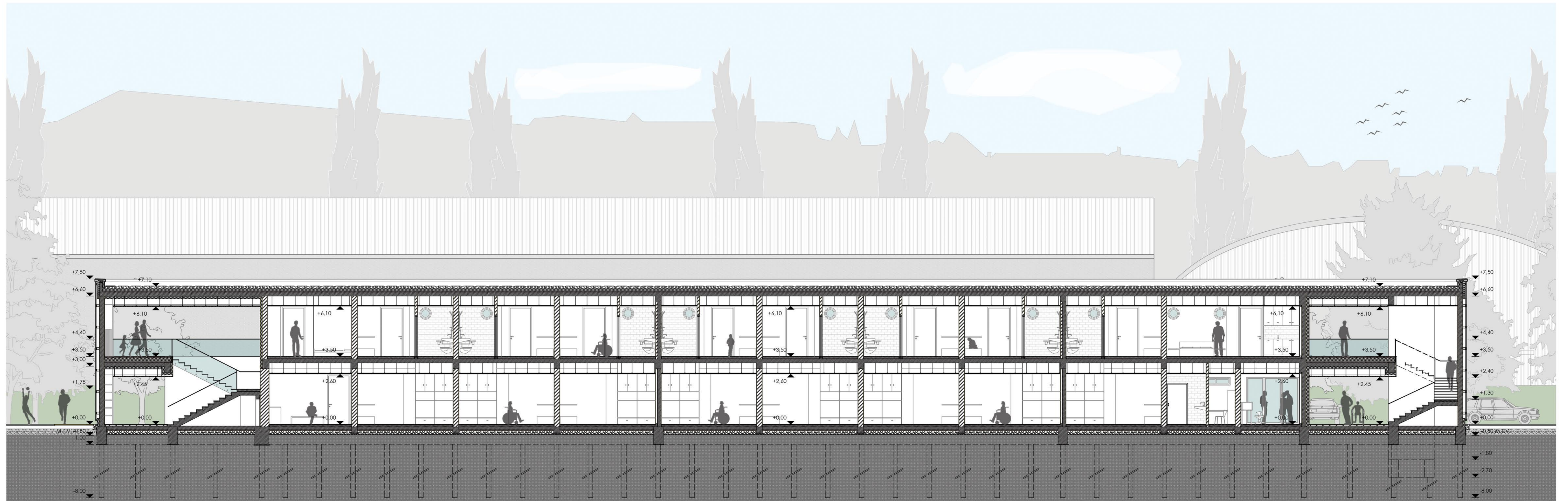
B-B metszet
