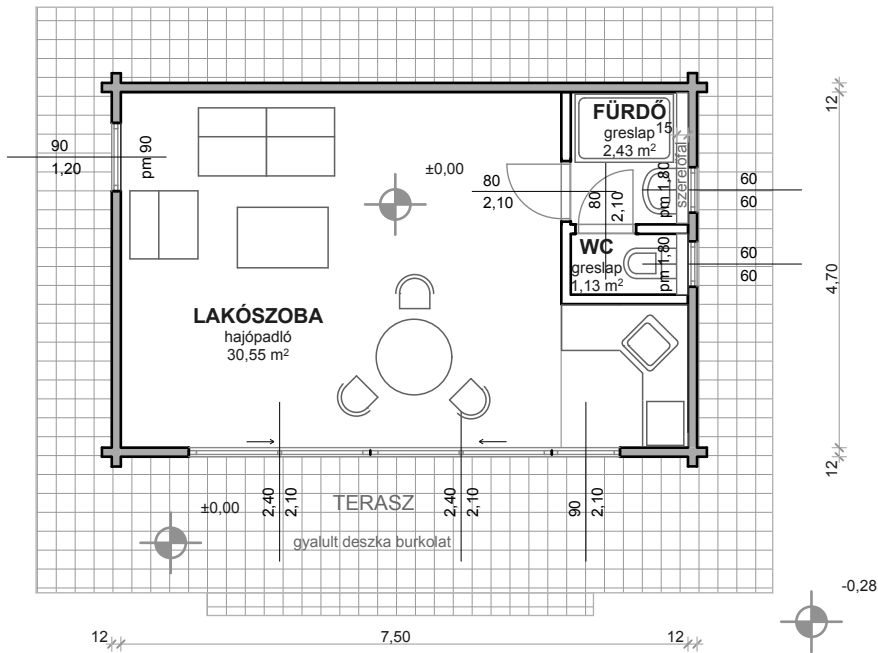
ALAPRAJZ
