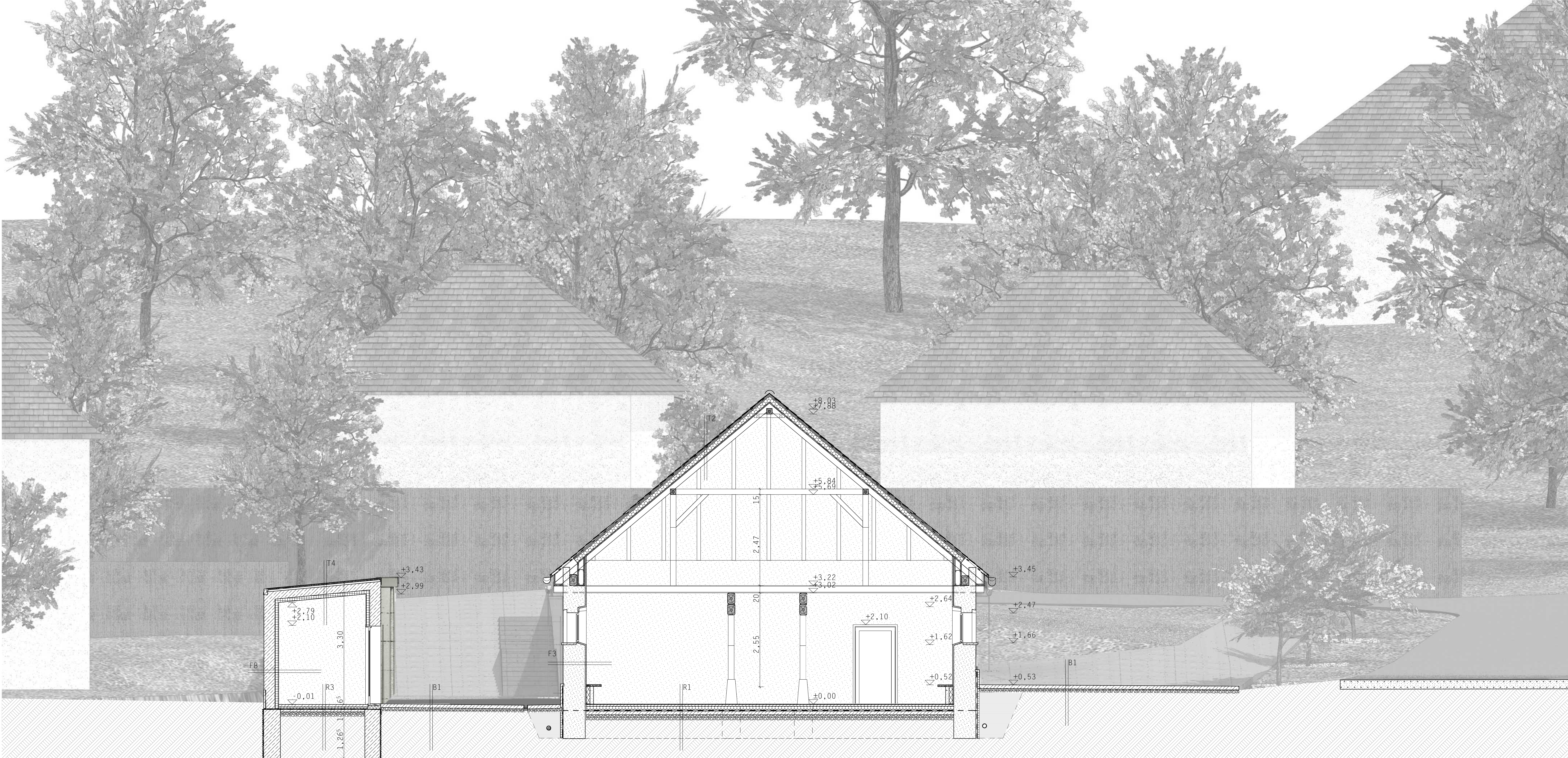
3-3 metszet m1:50
