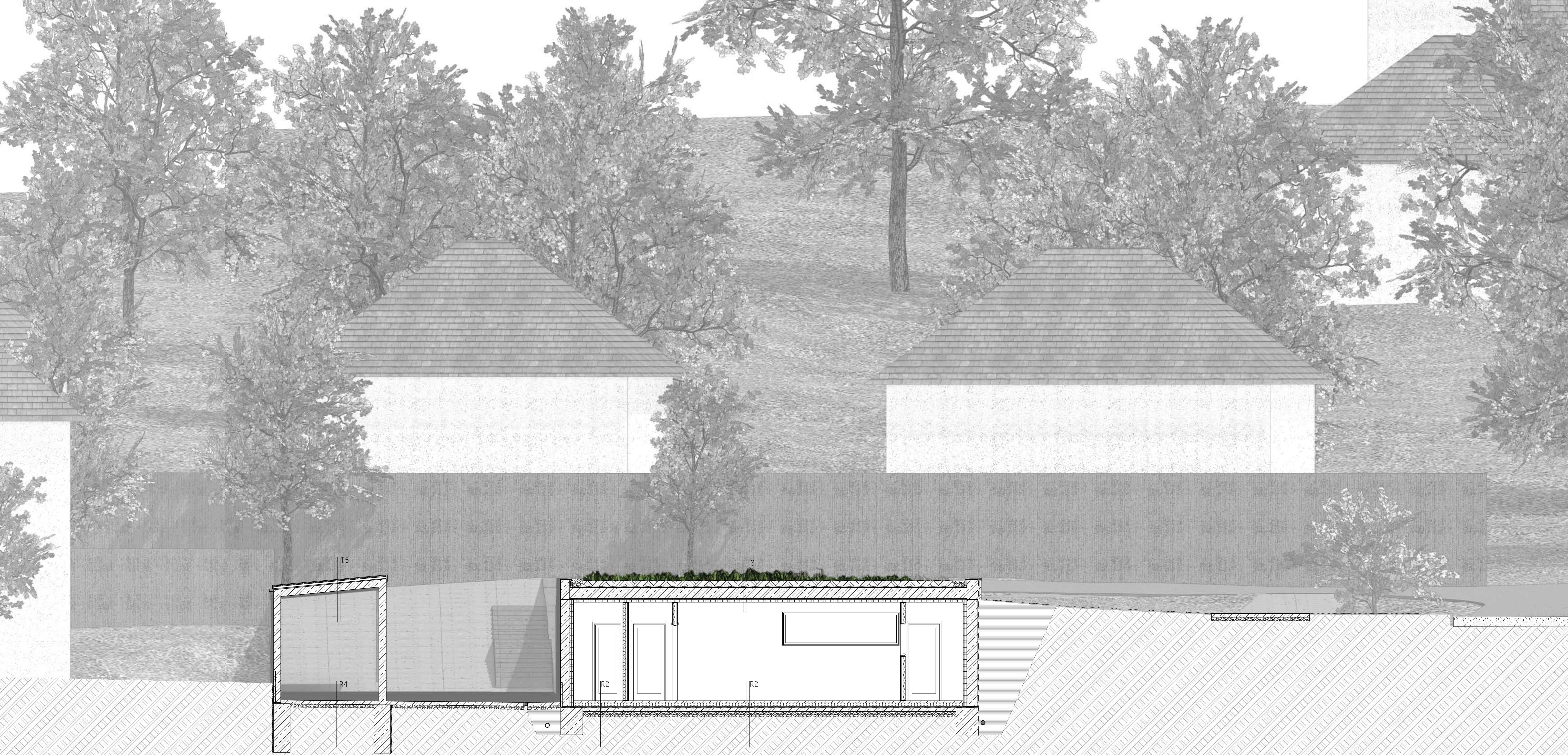
4-4 metszet m1:50
