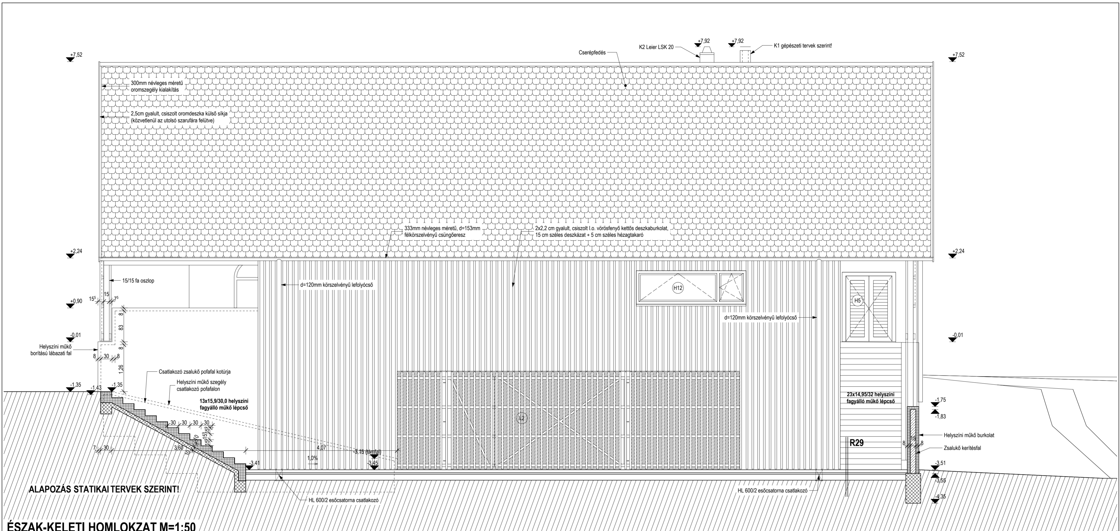
ÉSZAK-KELETI HOMLOKZAT M=1:50
